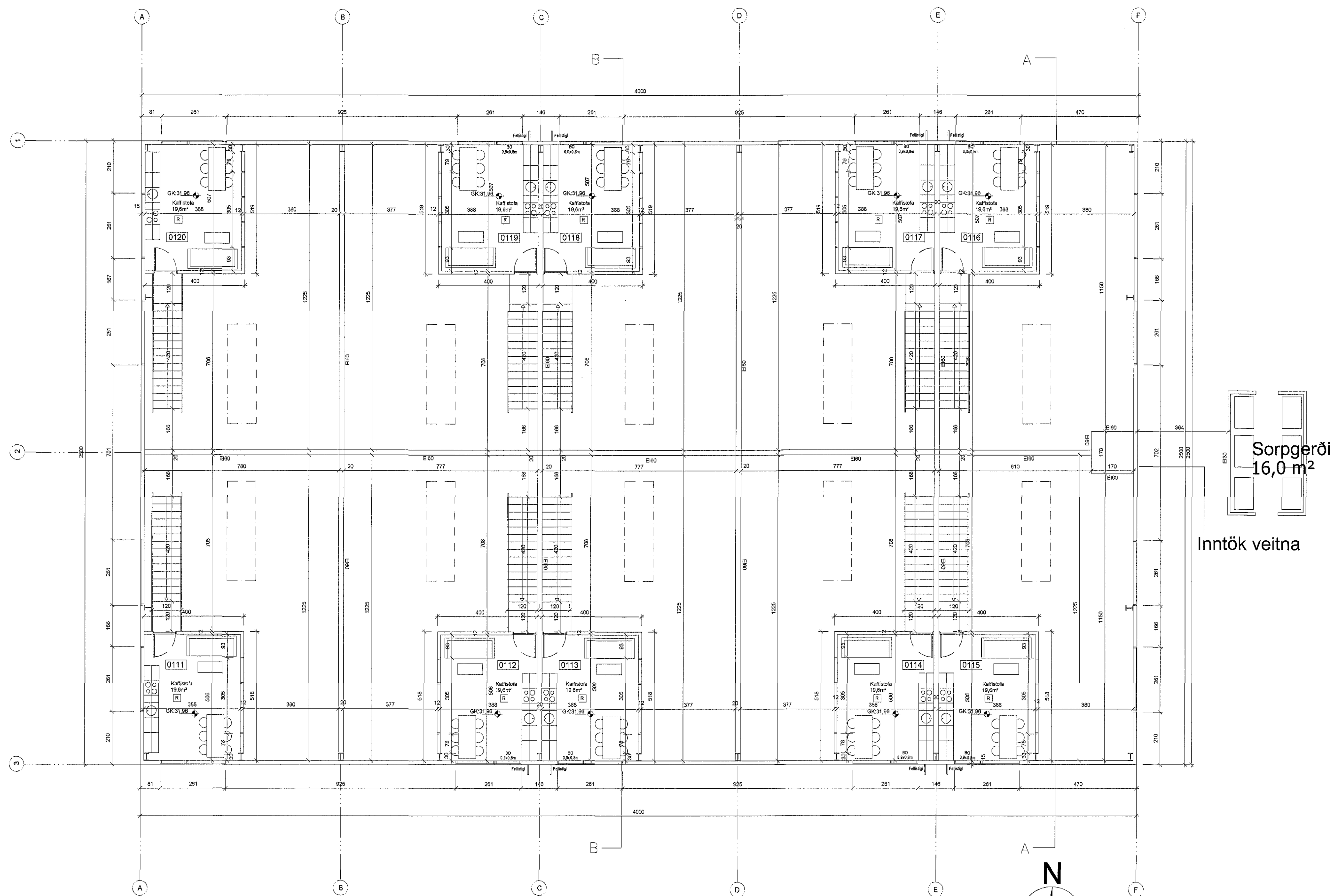
Grunnmynd 2. hæð 1:100
