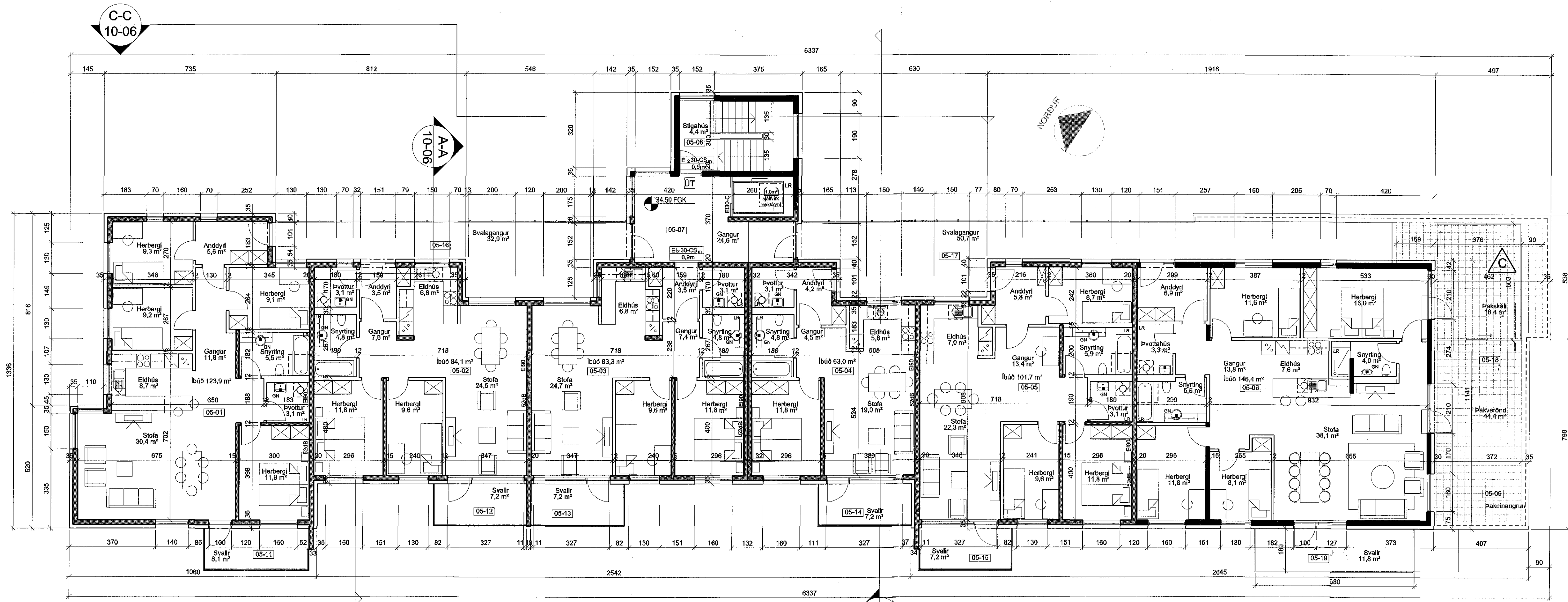
GRUNNMYND 1:100 5. HÆÐ
