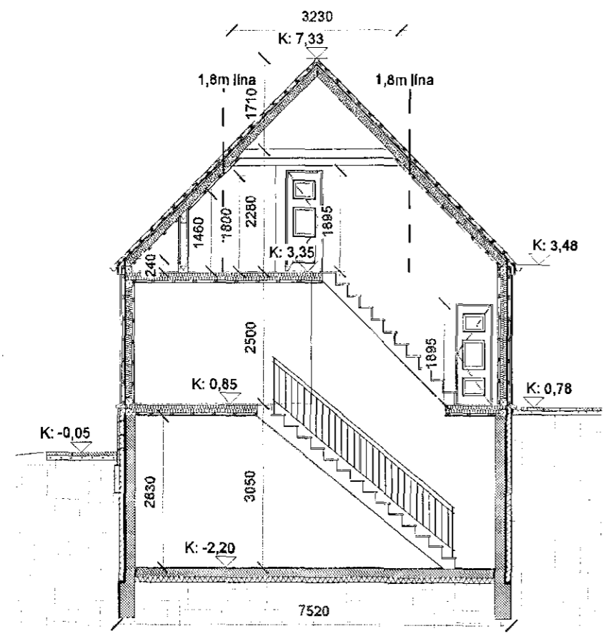
SNID A-A 1:100
