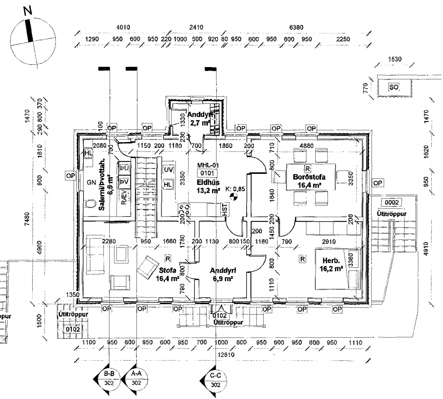
1. GRUNNMYND 1:100
