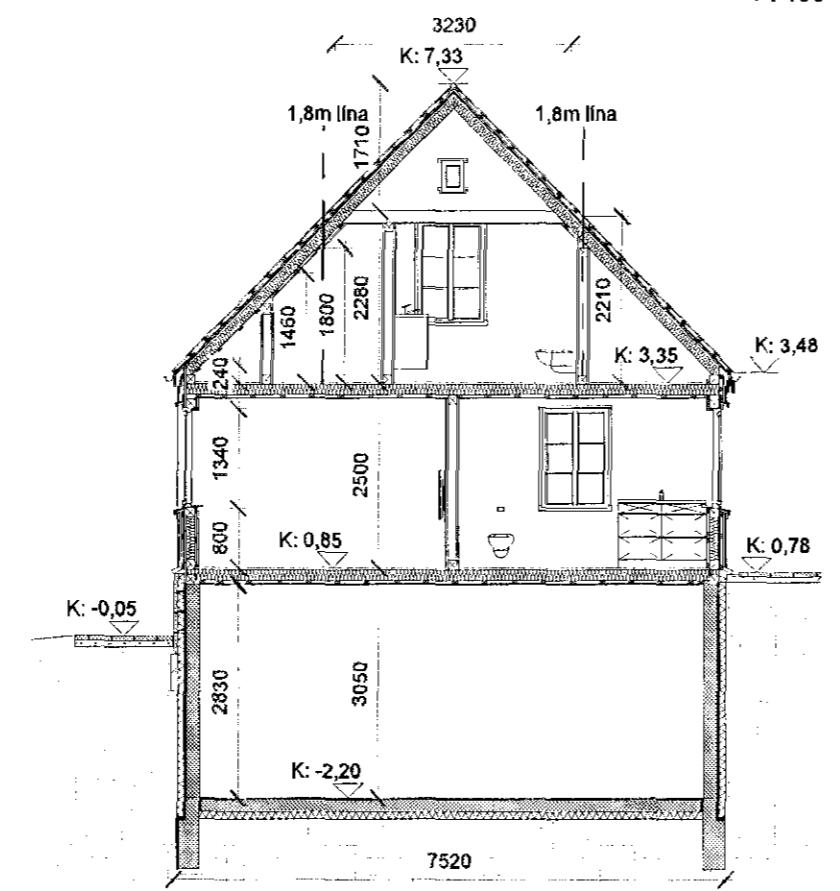
SNID B-B 1:100
