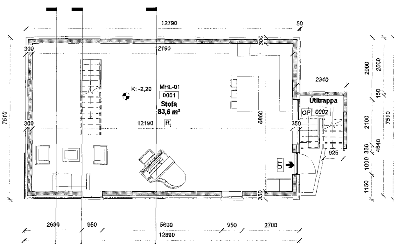
-1. KJALLARI 1:100
