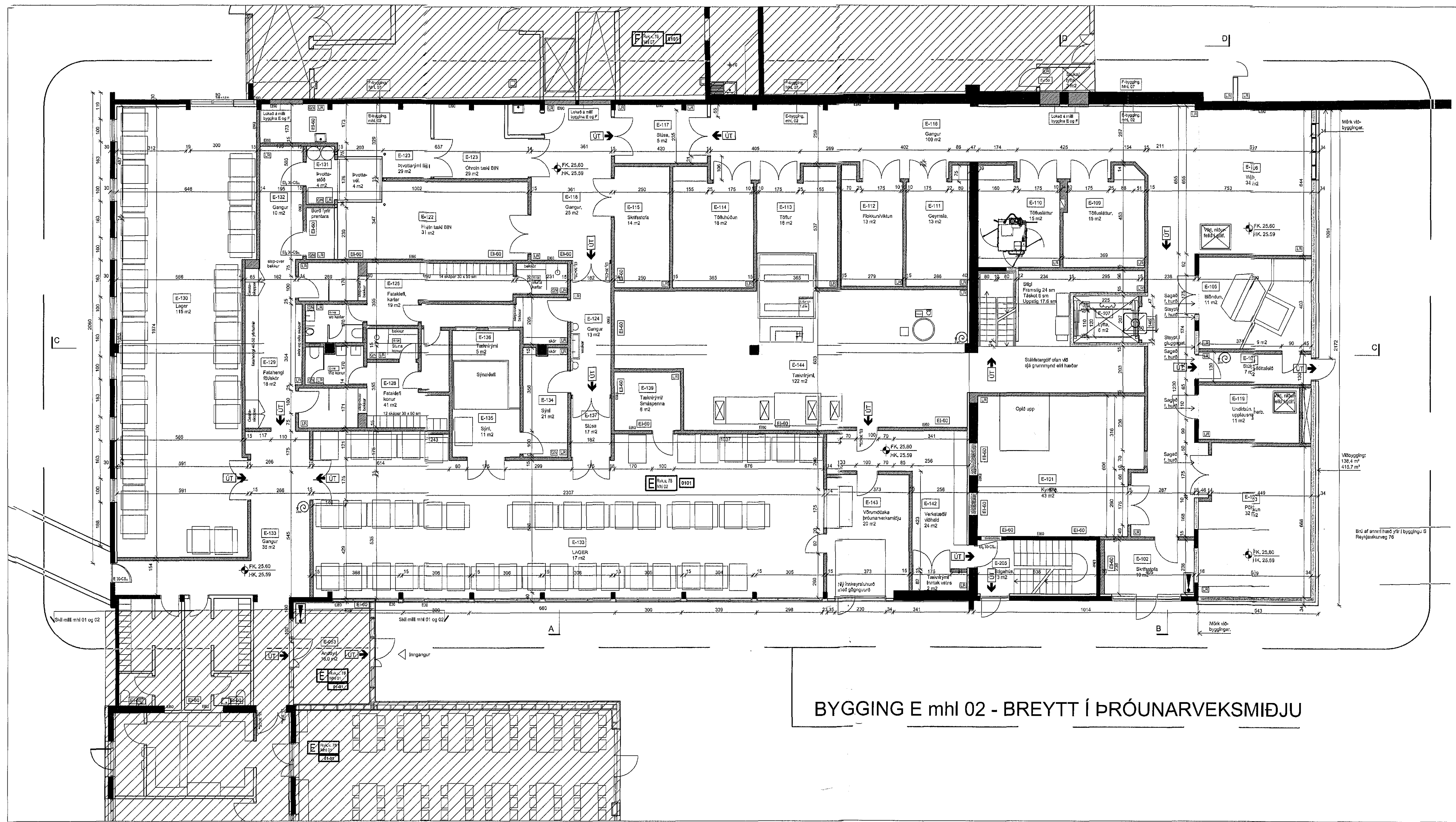
GRUNNMYND 1:100
