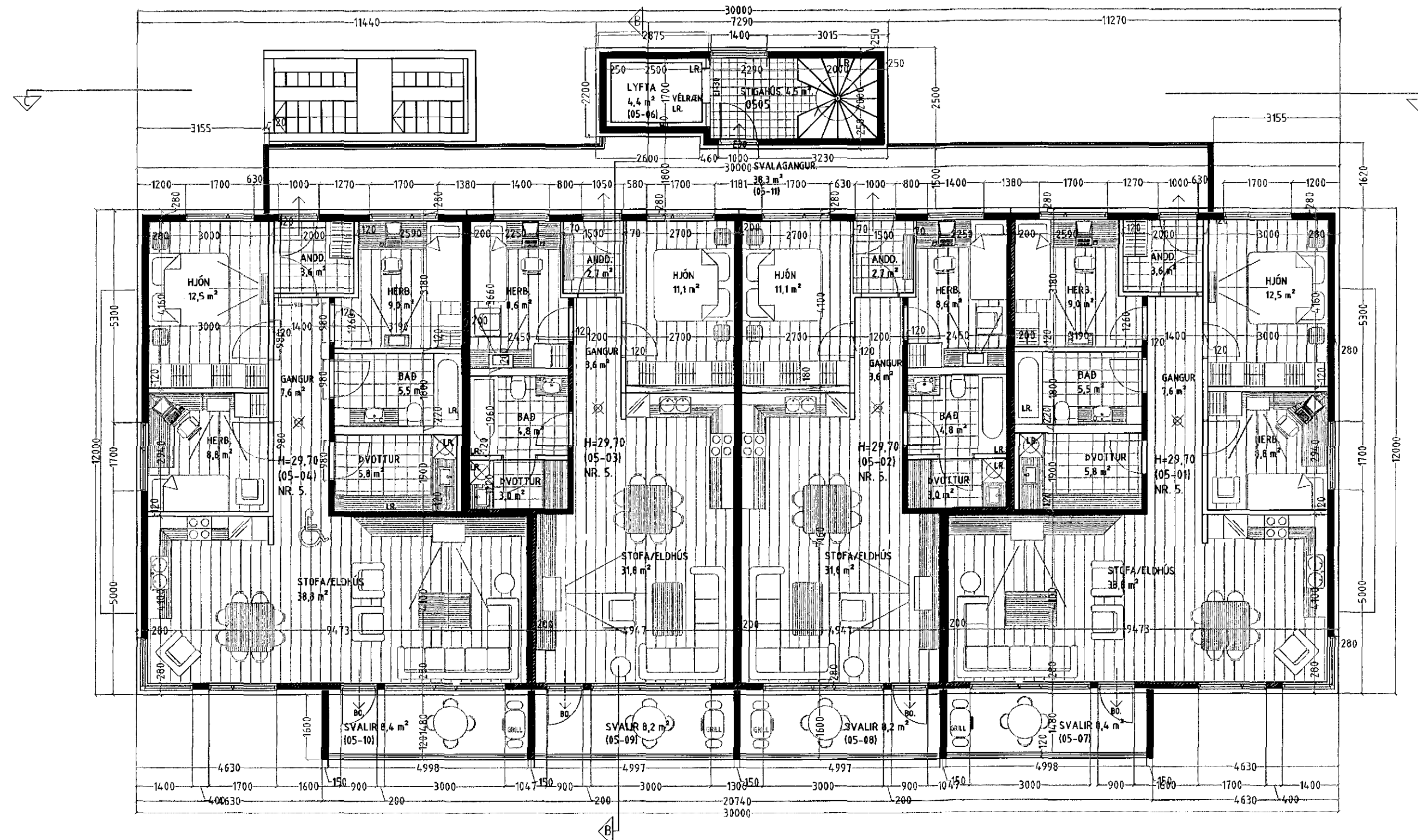
GRUNNMYND 5 HÆÐ. MKV. 1:100.
