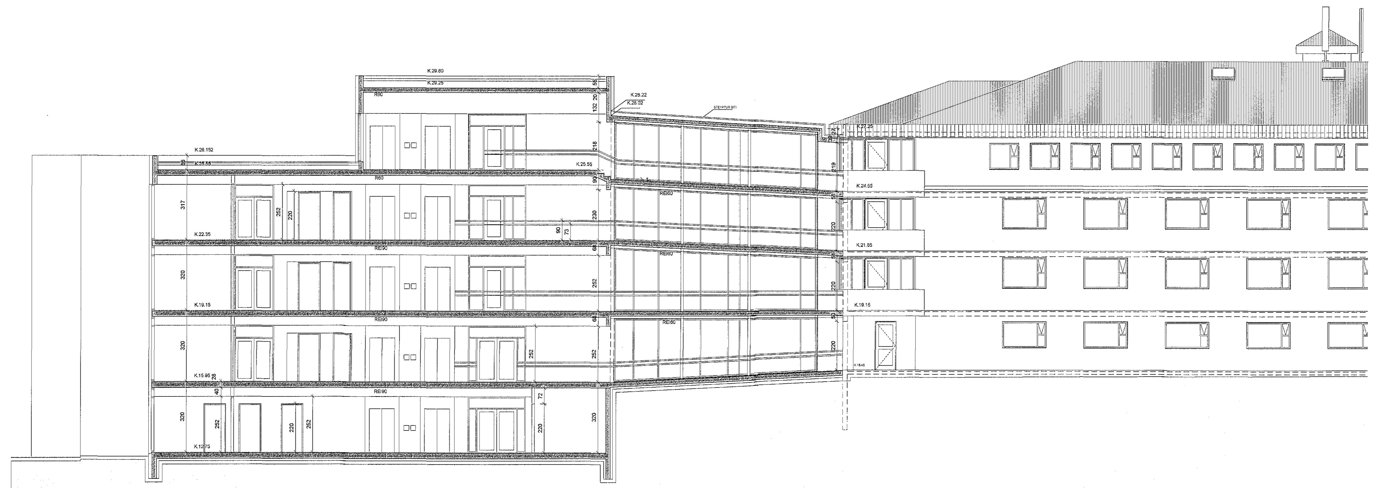
SNEIDING B-B 1:100
