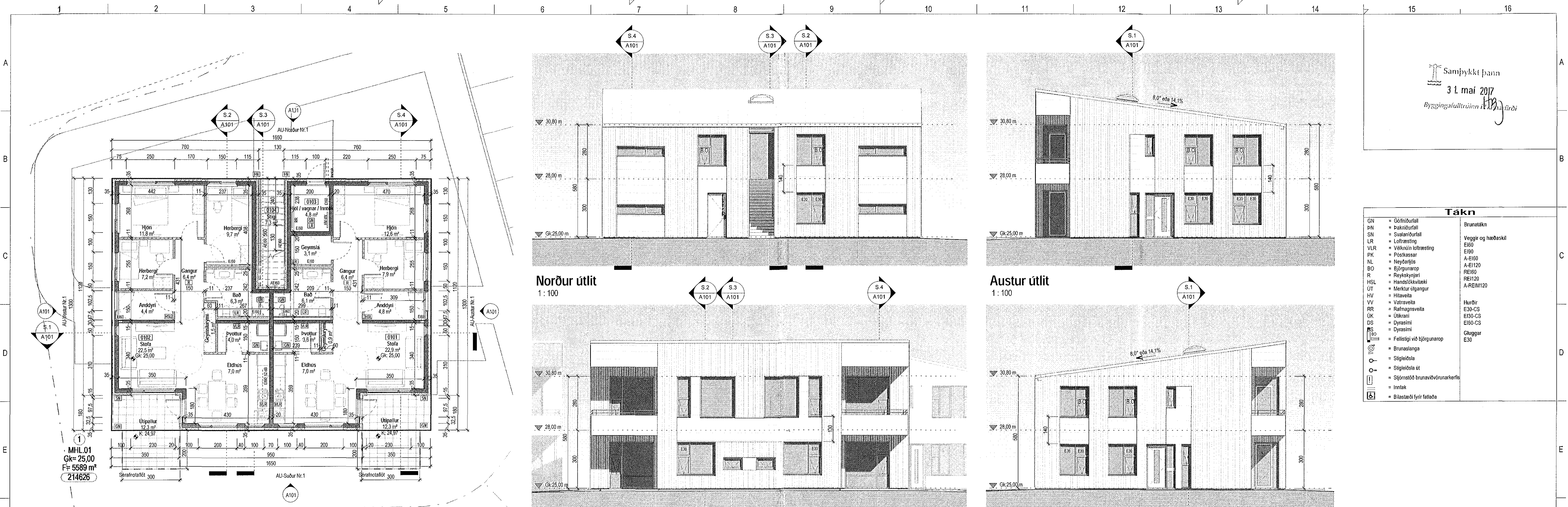
Grunnmynd 1. hæð 1:100
