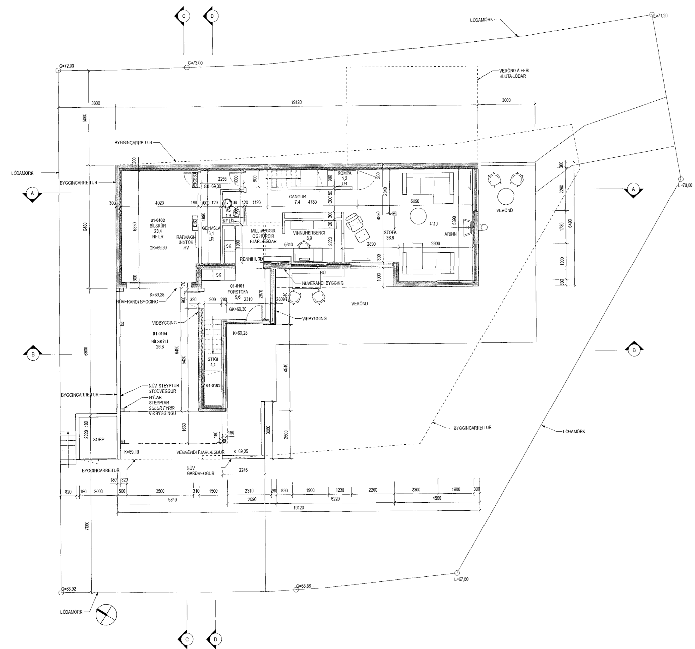
1 GRUNNMYND 1. HÆÐ 1:100
