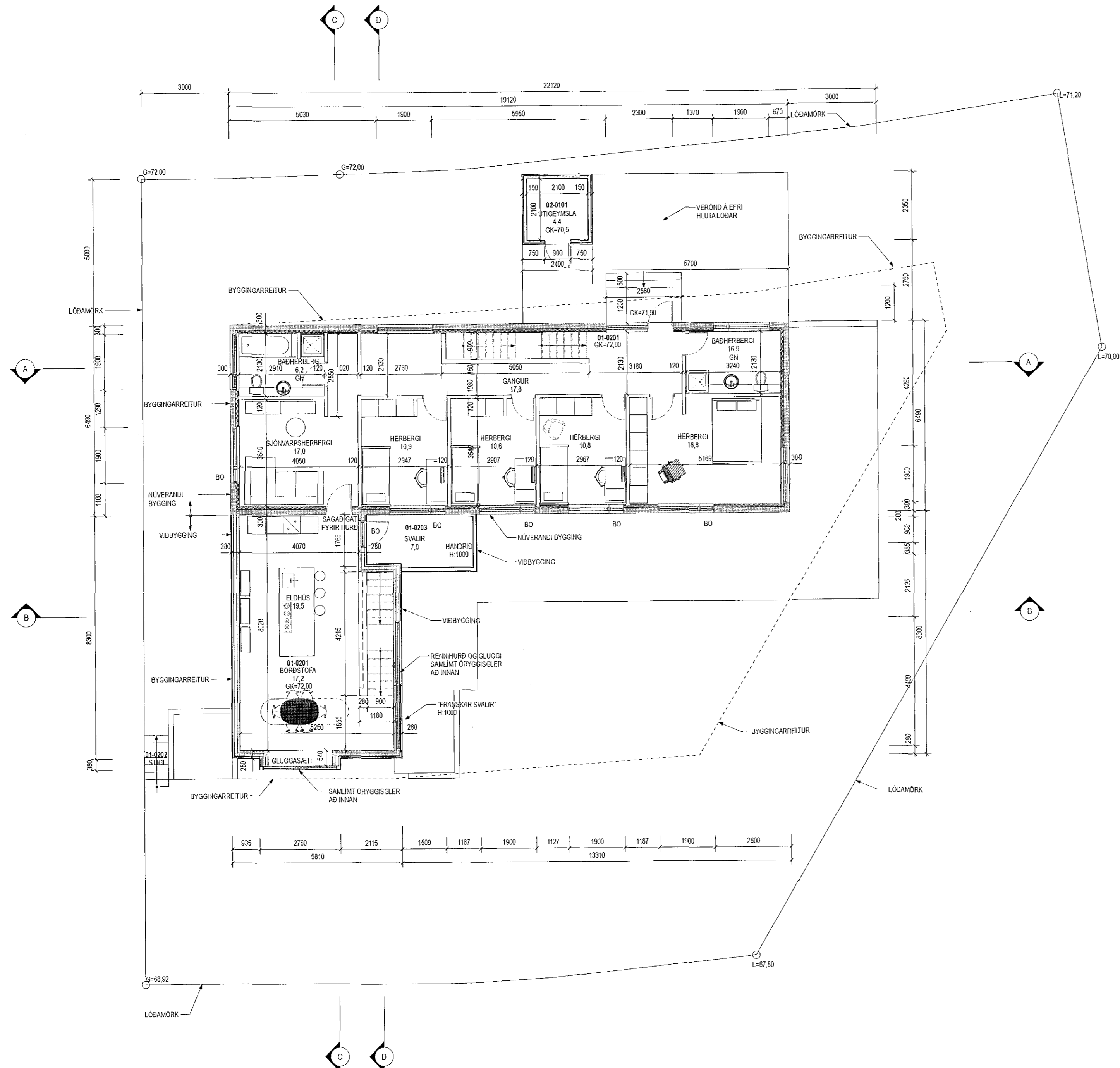
1 GRUNNMYND EFRI HÆÐAR 1:100
