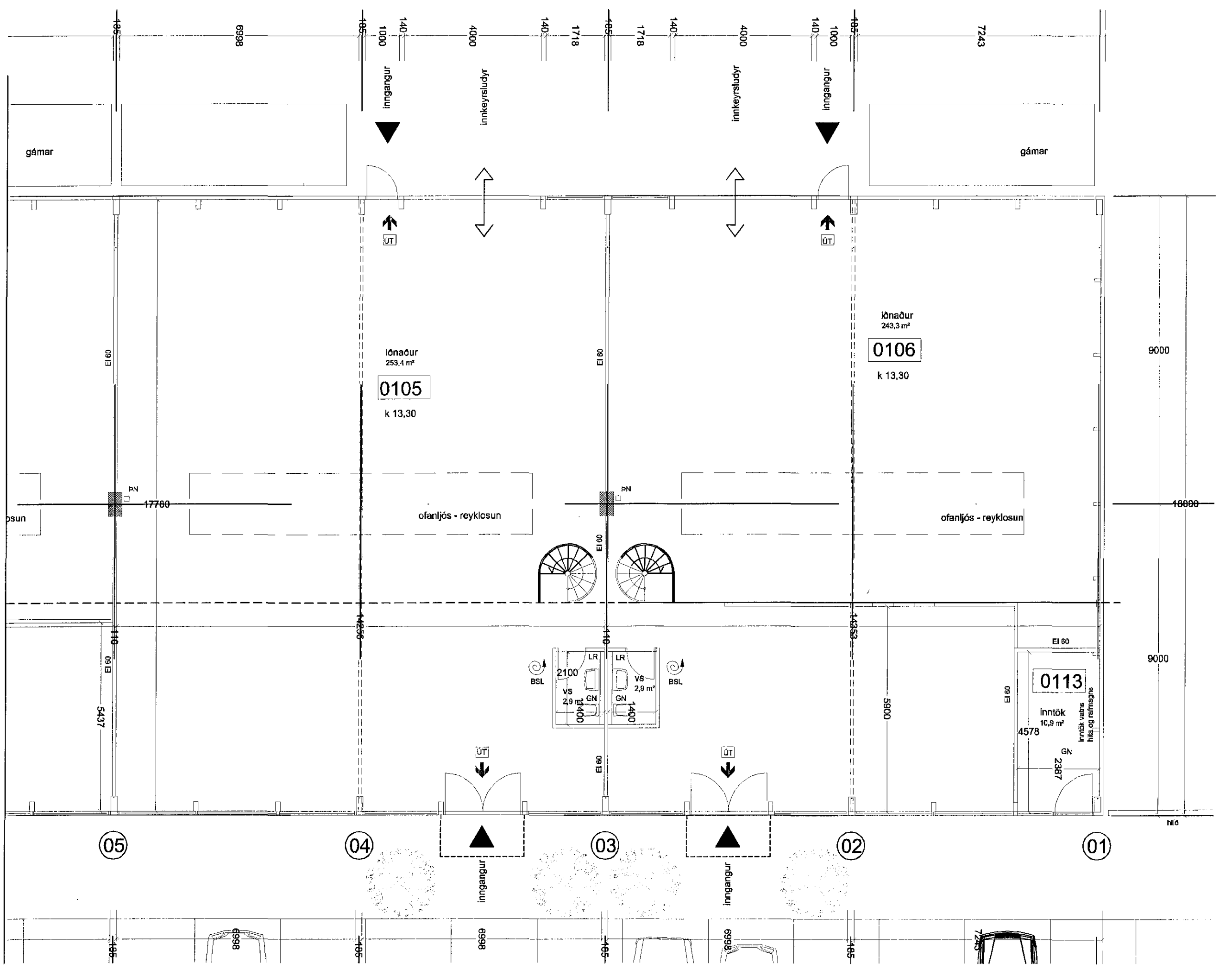
GRUNNMYND, 1.HÆÐ - 2.HLUTI MKV 1:100
