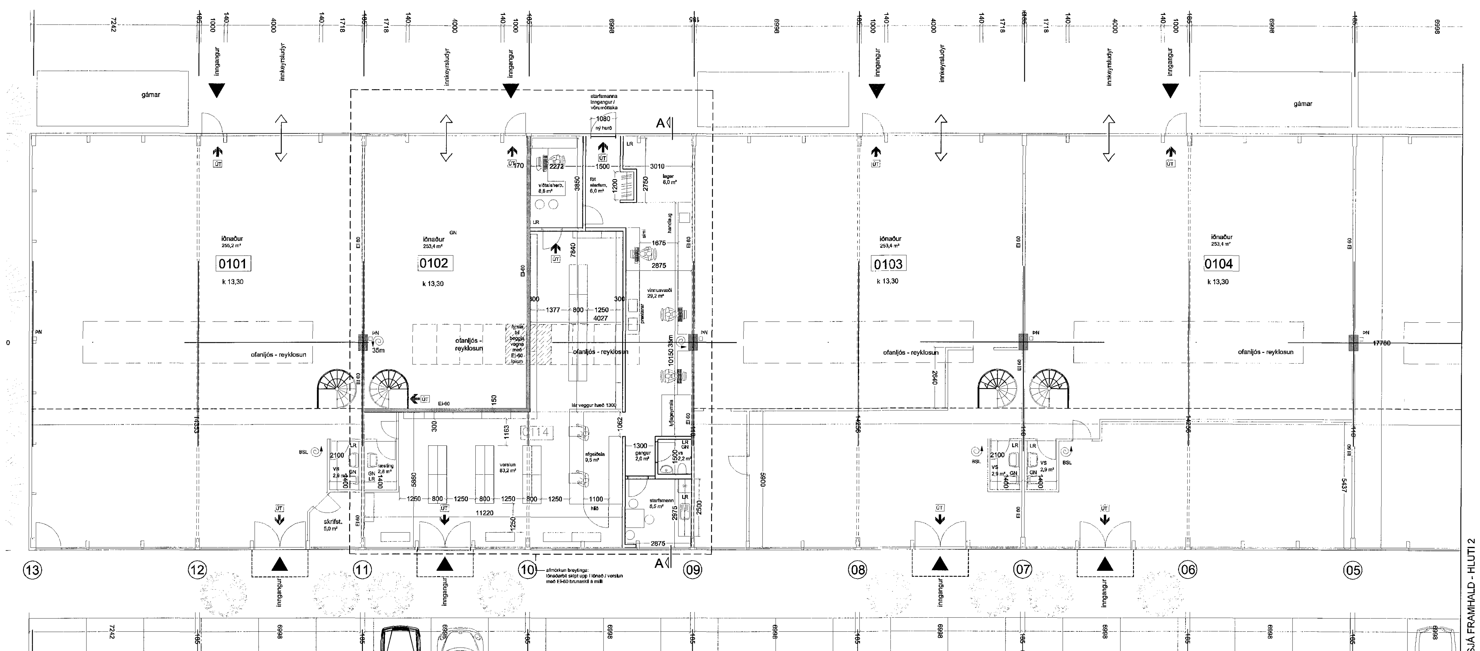
GRUNNMYND, 1.HÆÐ - 1.HLUTI MKV 1:100
