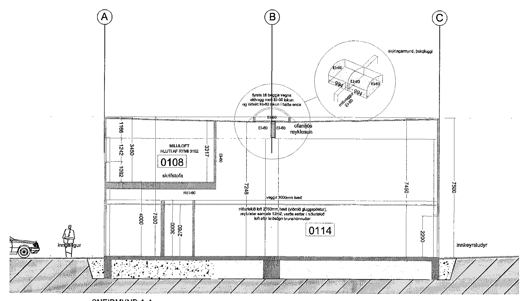
SNEIÐMYND A-A MKV 1:100
