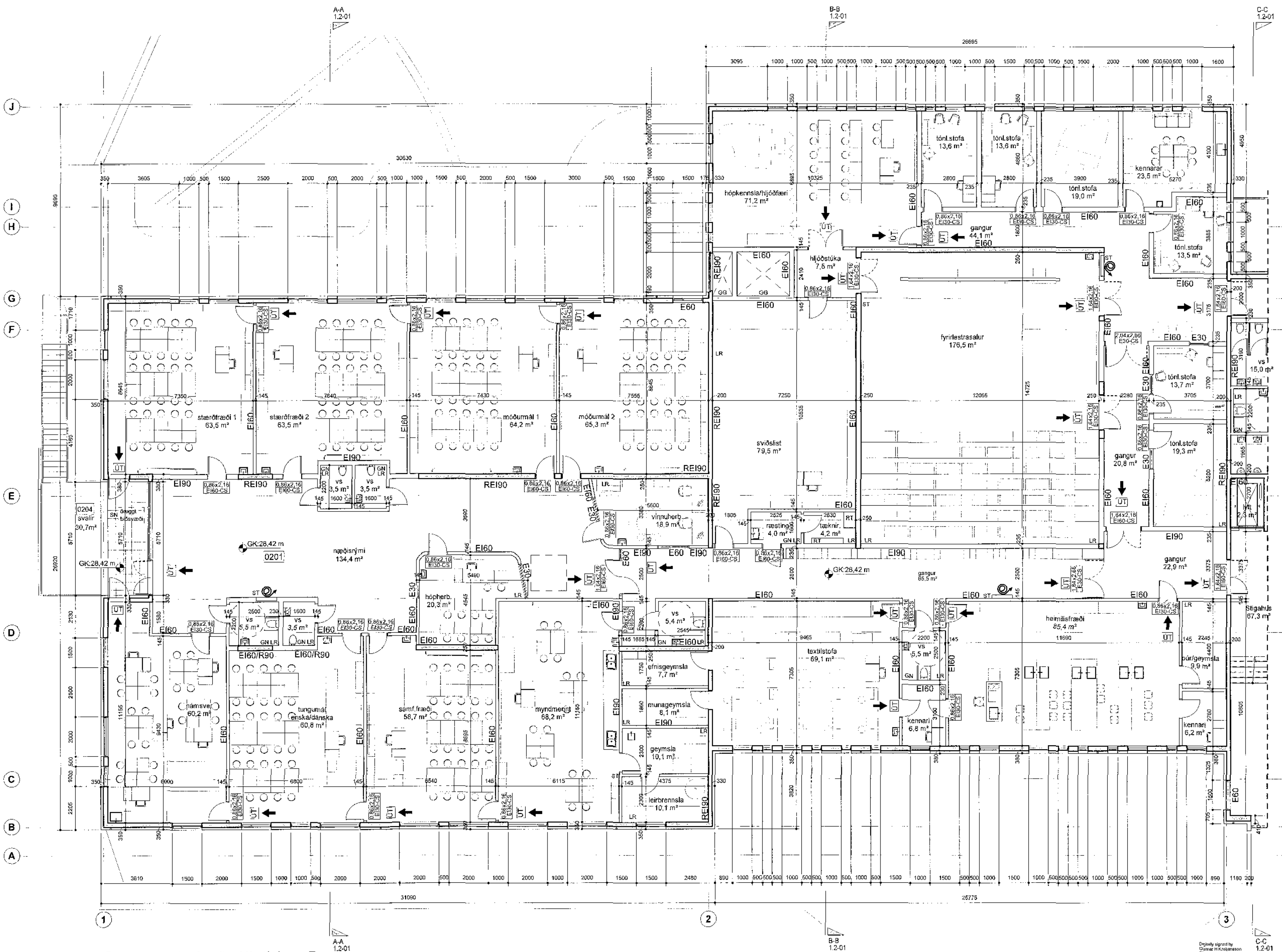
Grunnmynd 2.hæð - Hluti A og B mkv. 1: 100
