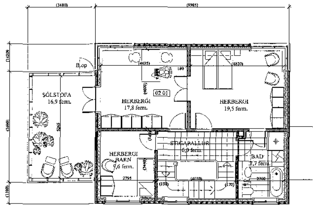
GRUNNMYND KJALLARA
