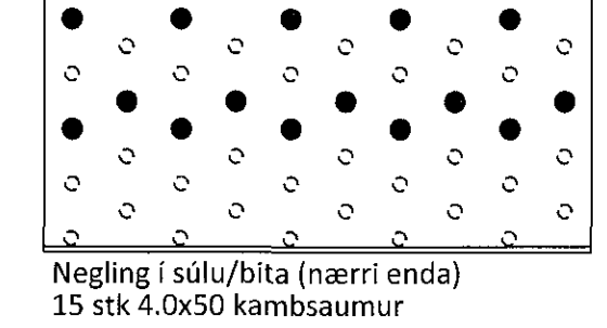
X - BMF-65x95x2.5x200 vinklar
