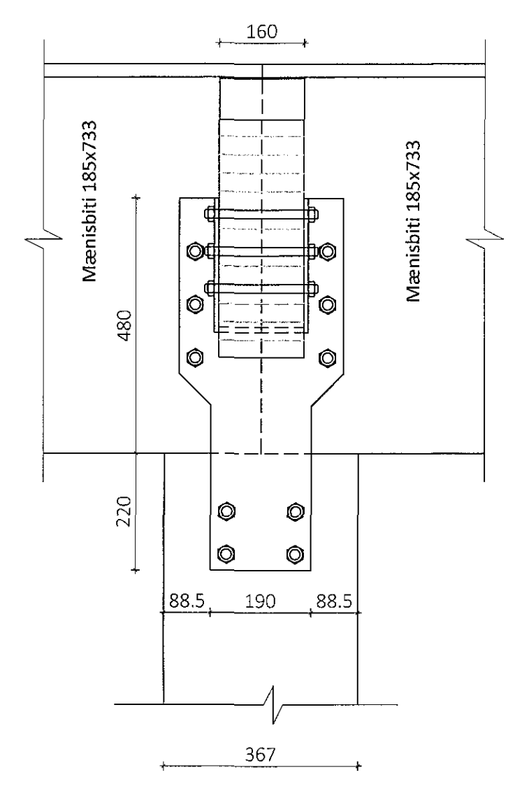
Snið A-A
