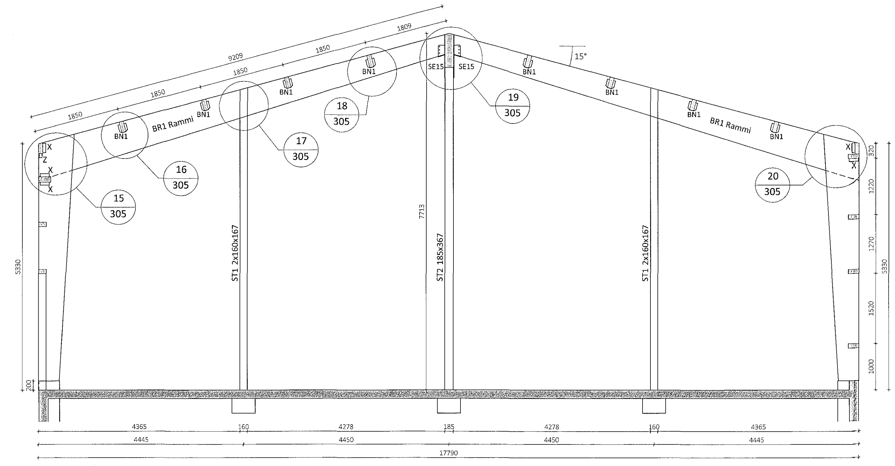
pversnið A-A Mkv. 1:50
