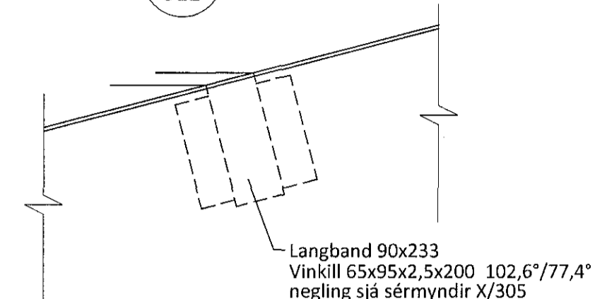
Sérmynd 45 Mkv. 1:10 312
