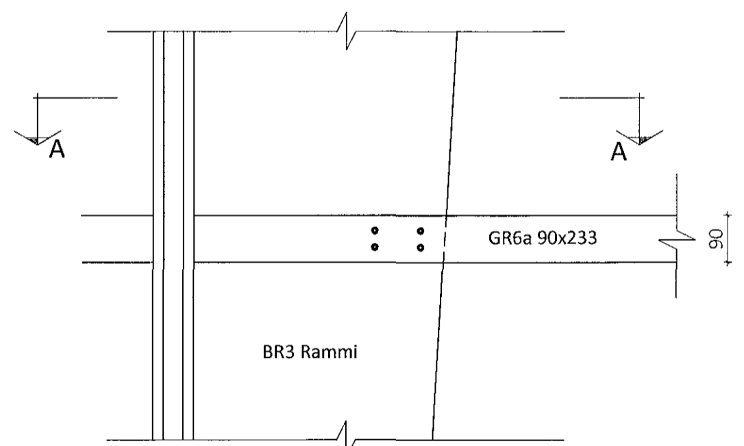
Sérmynd 42 Mkv. 1:10 312
