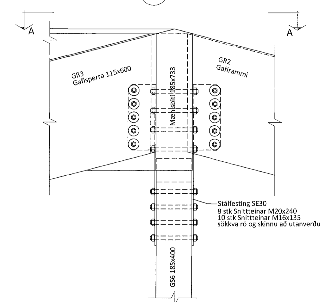
Sérmynd 46 Mkv. 1:10 312
