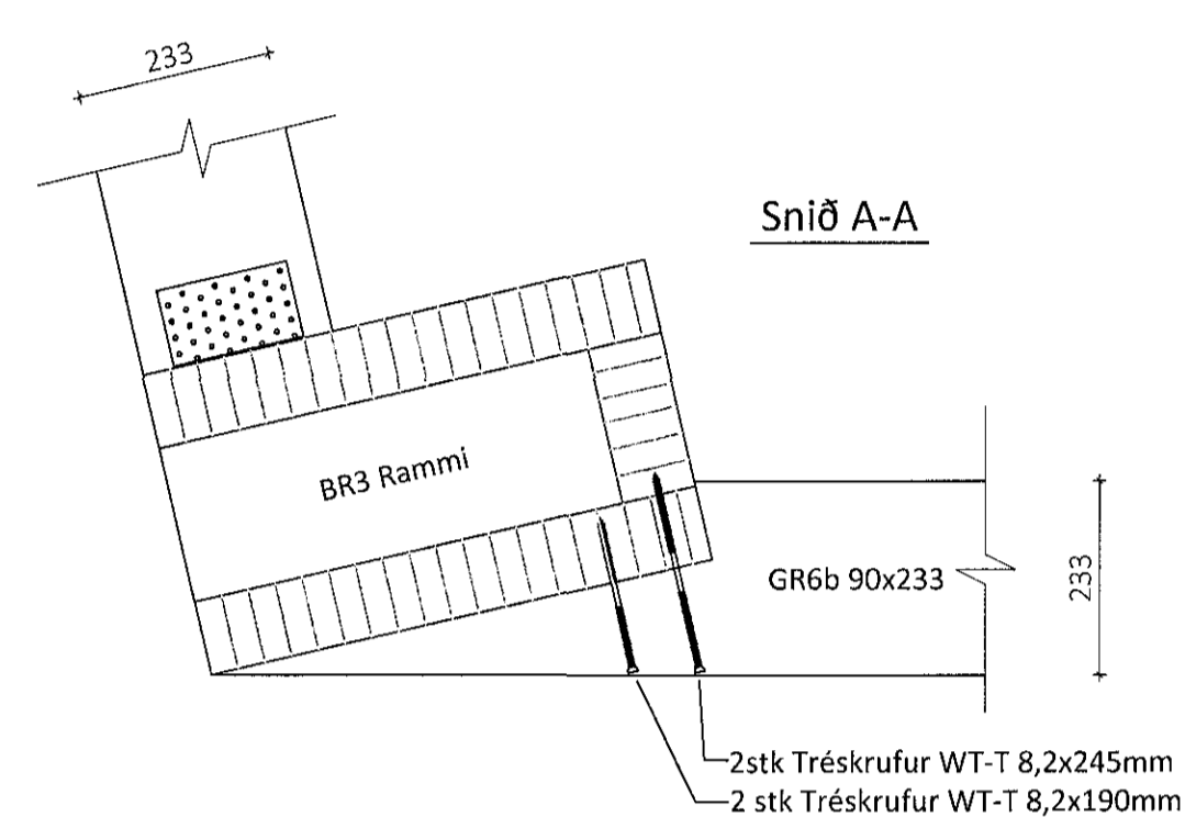
Sérmynd 42 Mkv. 1:10 312
