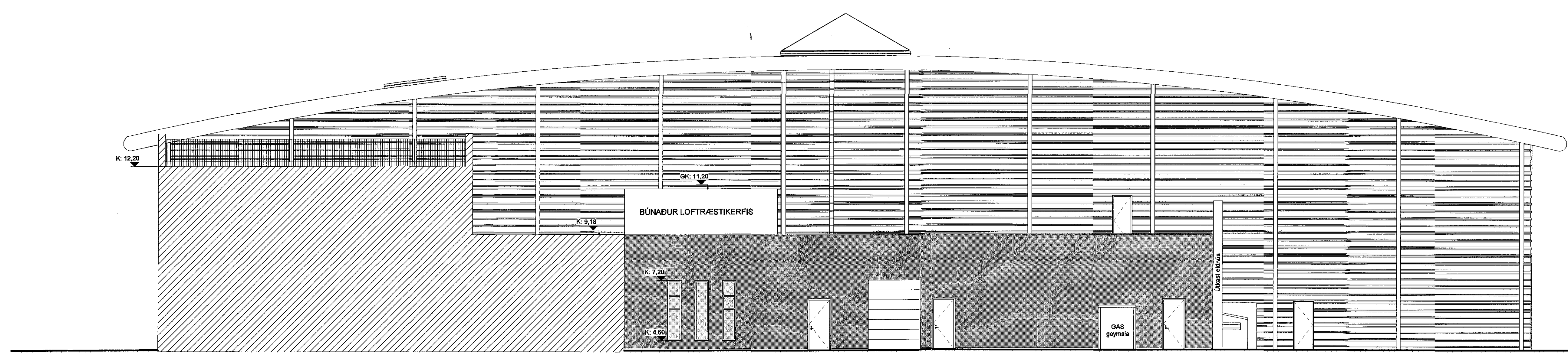
ÚTLIT AUSTUR BAKHÚS
