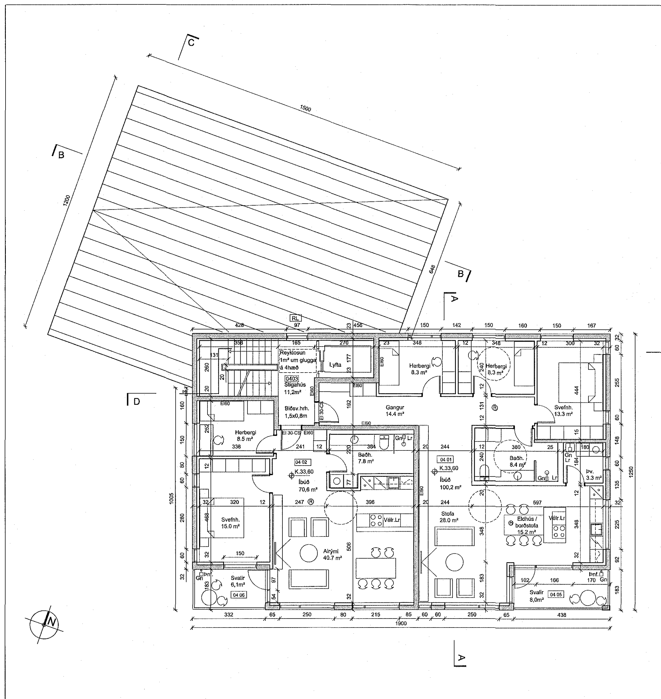
GRUNNMYND 4 HÆÐ
