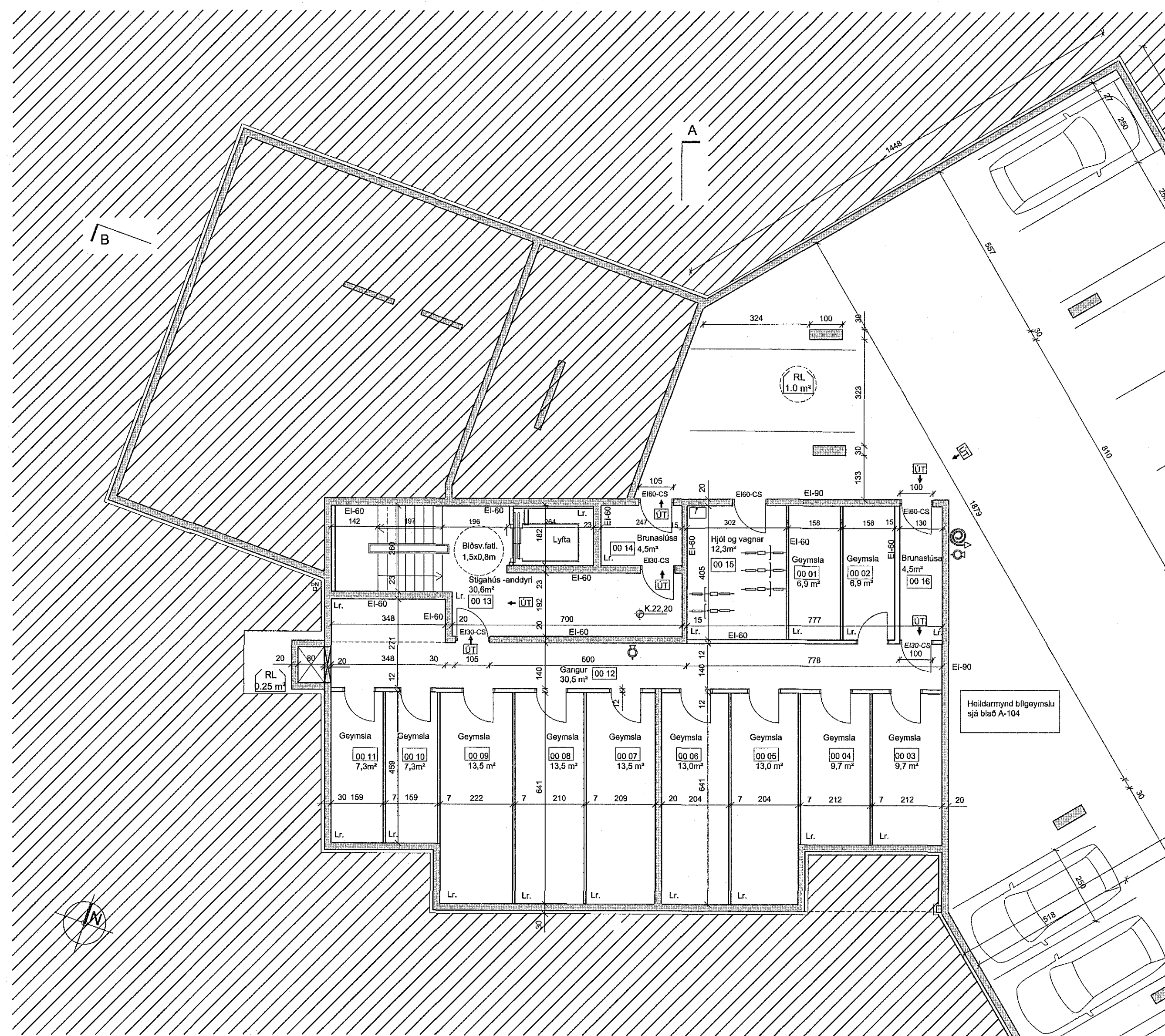
GRUNNMYND KJALLARI - GEISLASKARÐ. 4 MKV 1:100
