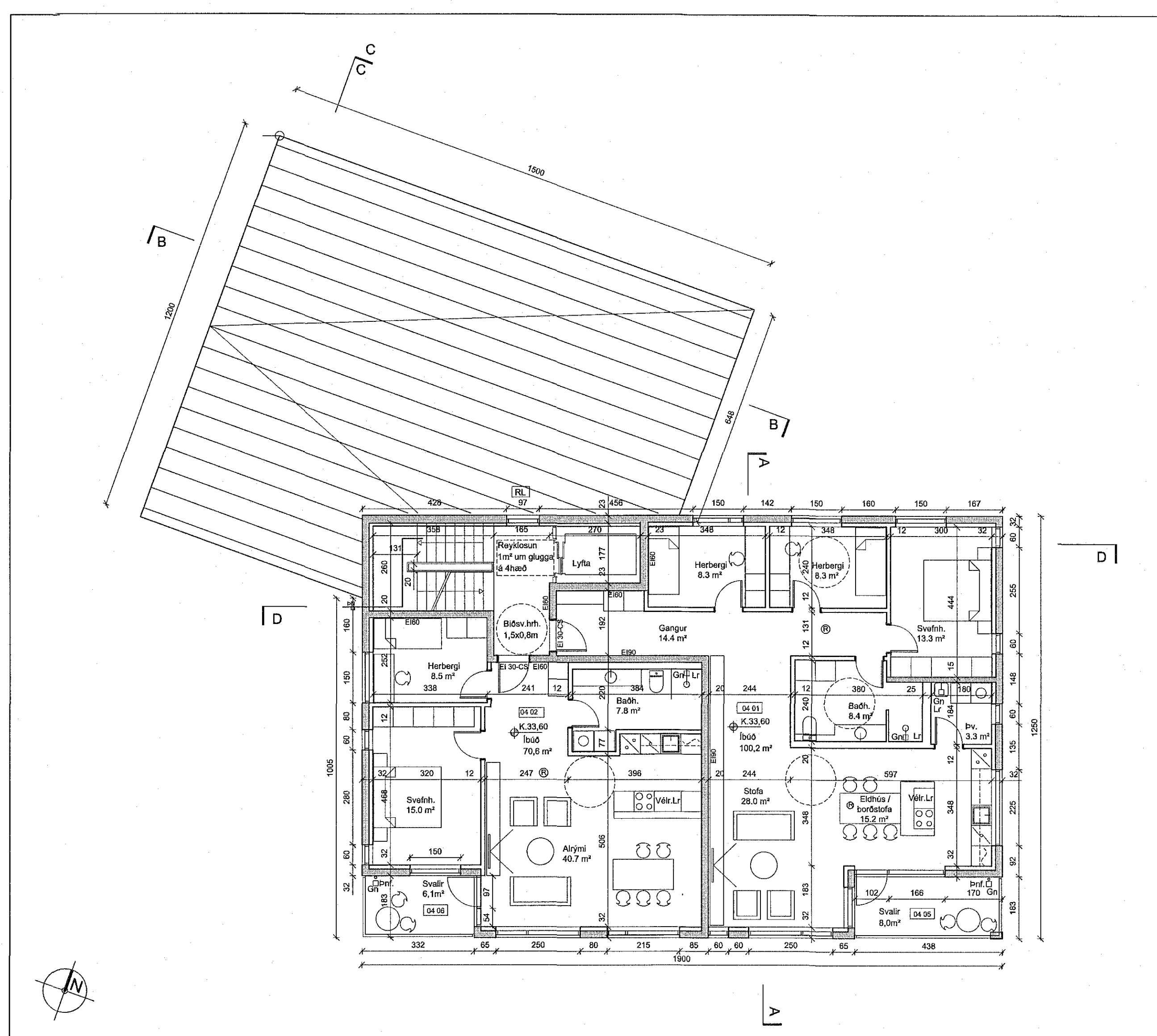
GRUNNMYND 4 HÆÐ
