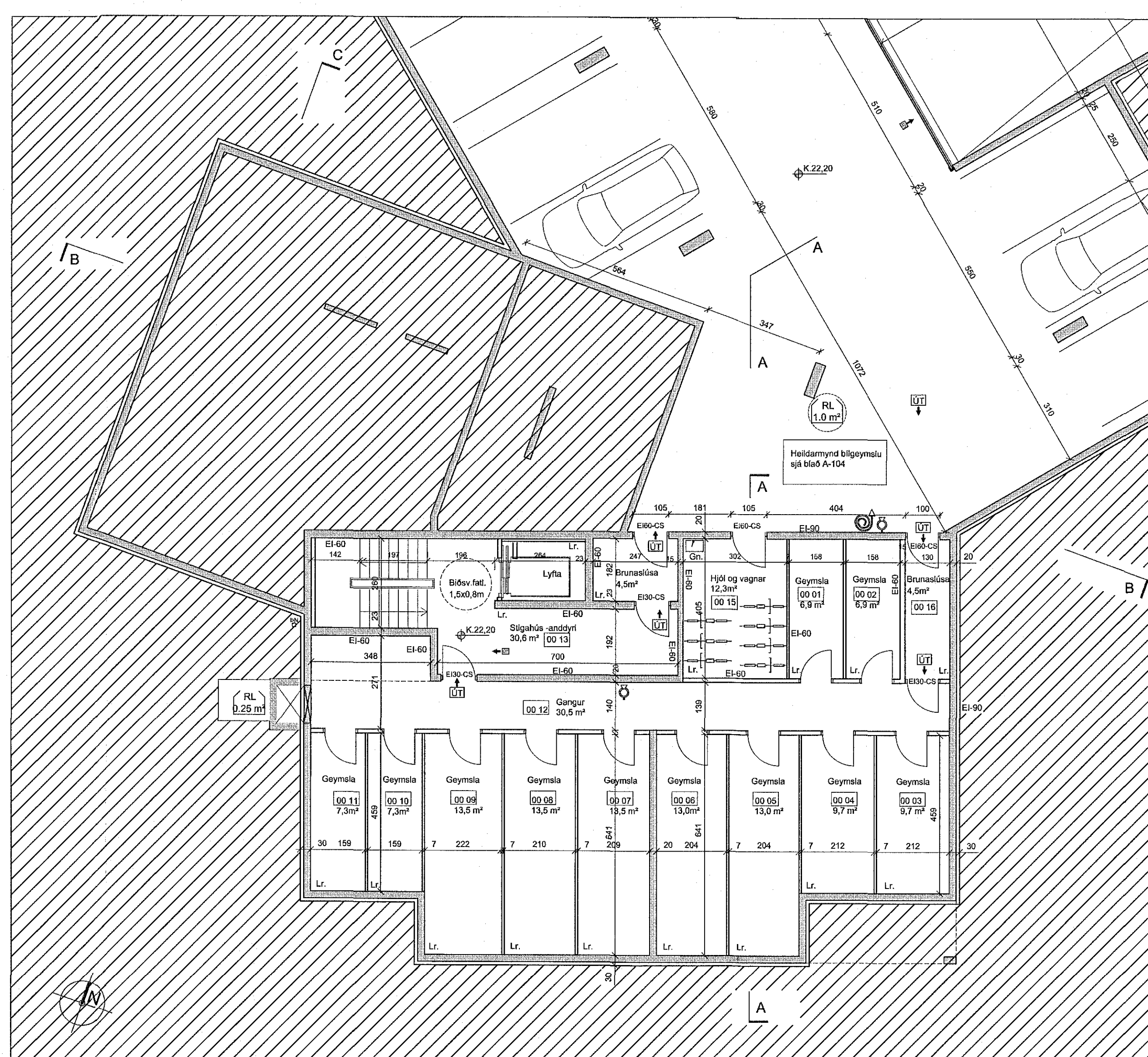
GRUNNMYND KJALLARI MKV 1:100
