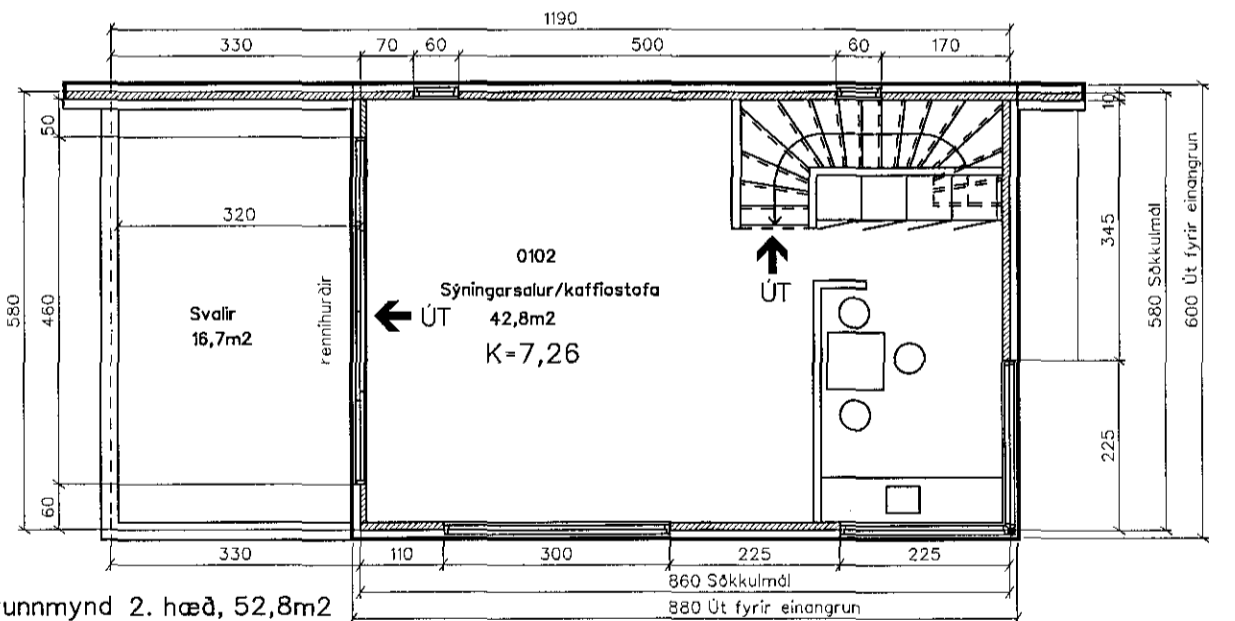
Grunnmynd 2. hæð, 52,8m2
