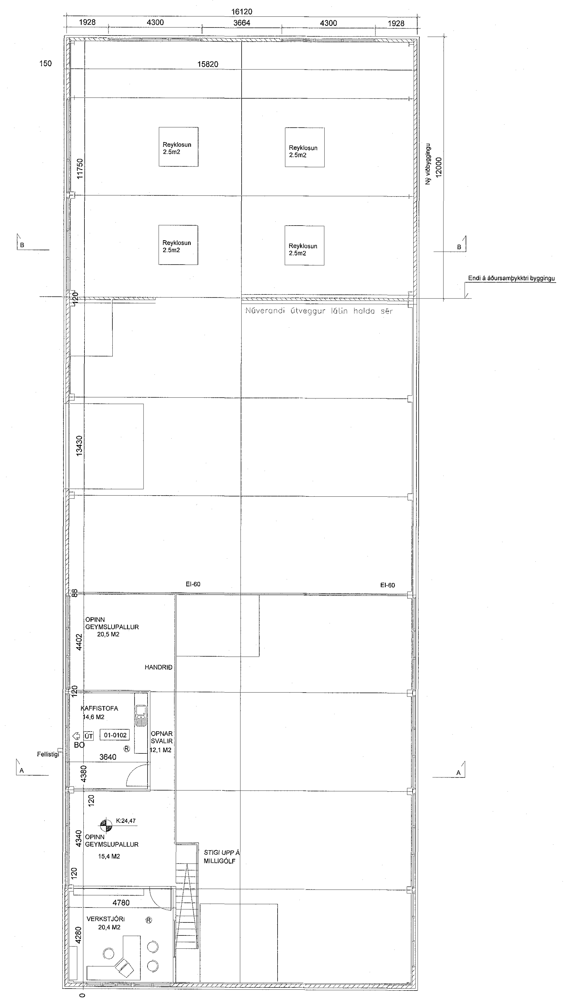
GRUNNMYND 2. HÆÐ, 1:100
