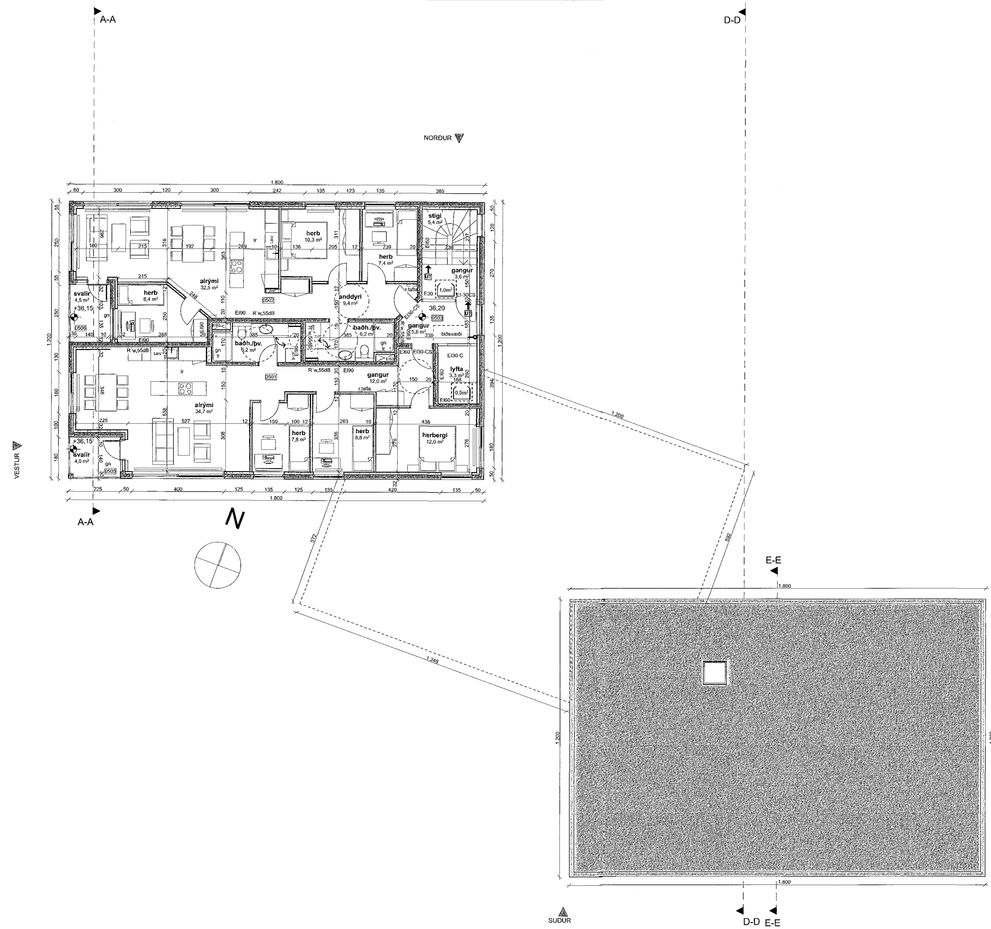
5. Hæð
