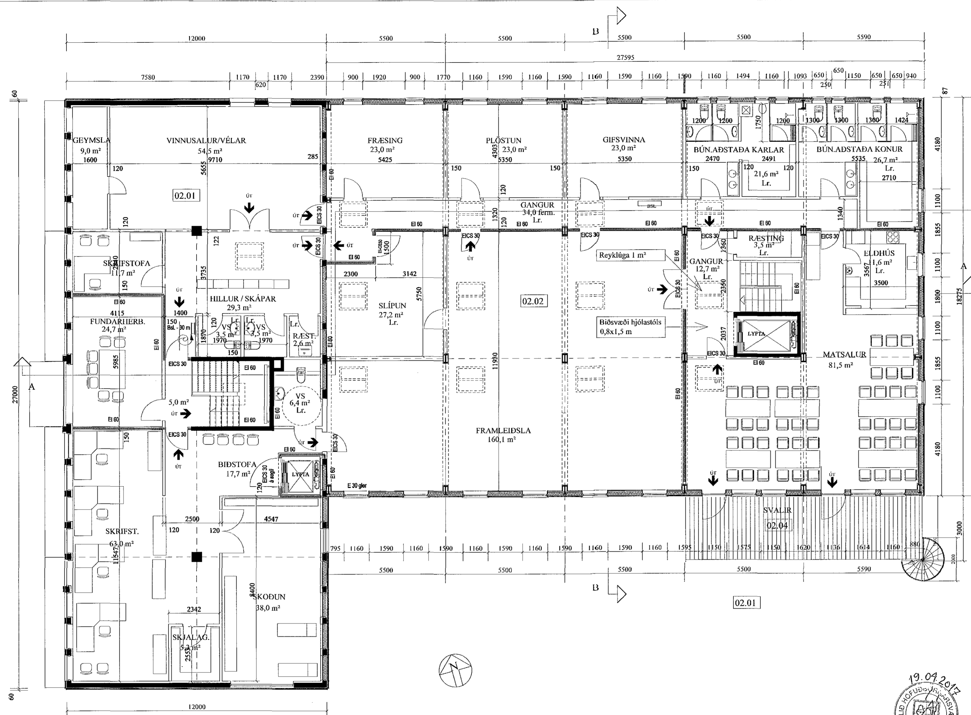
GRUNNMYND 2. HÆÐ
