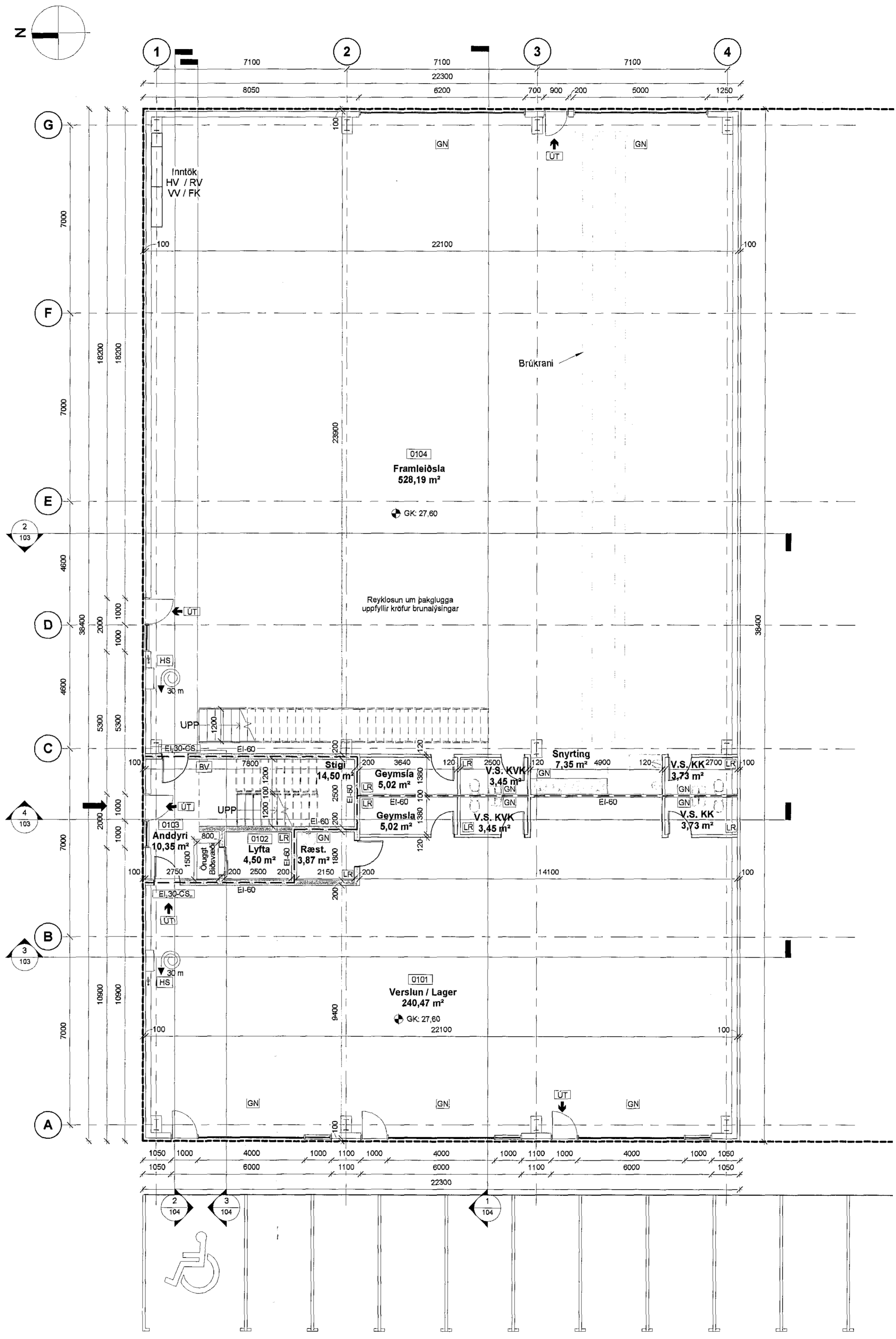
1 1. Hæð 1:100
