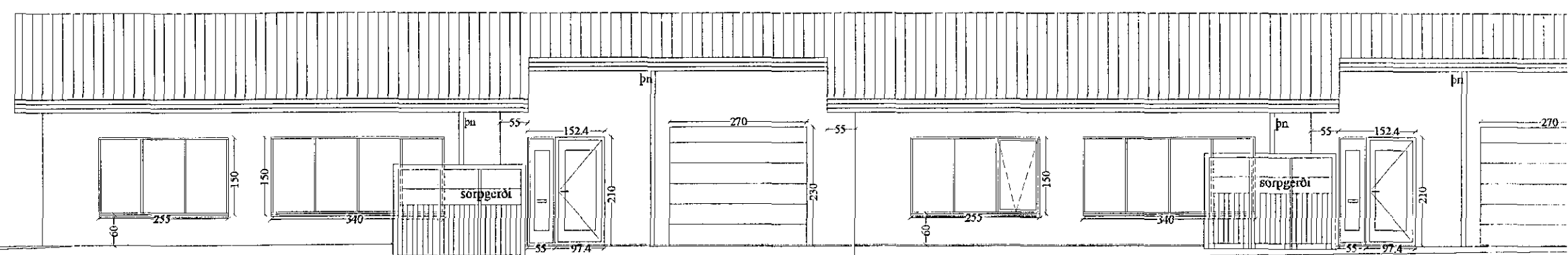
útlit norður hús nr. 35 mkv.: 1:100
