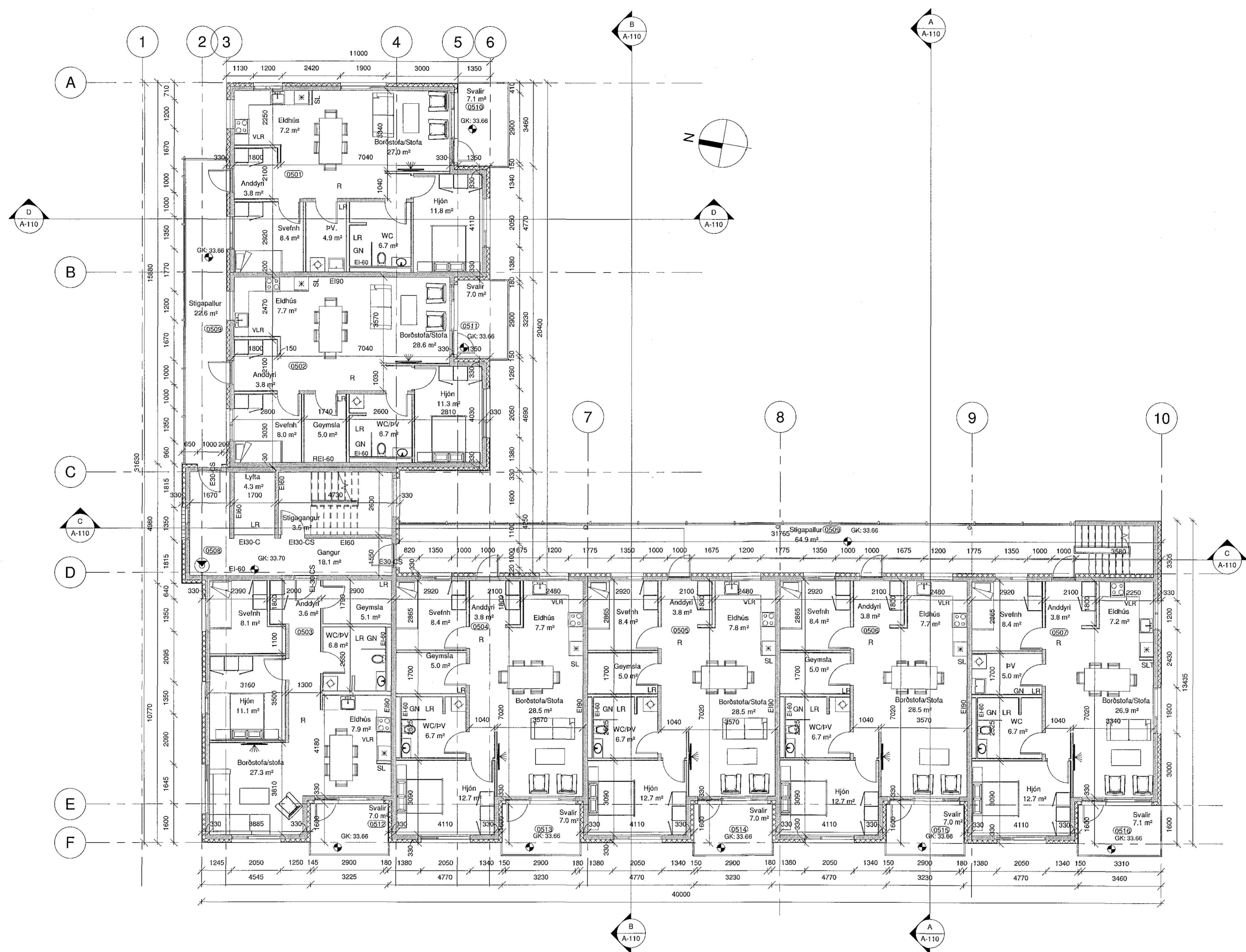
1 5.Hæð 1 : 100
