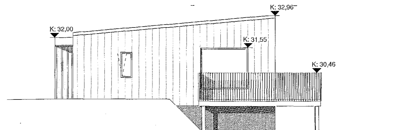
mhl. 04 ásýnd austur 1:100
