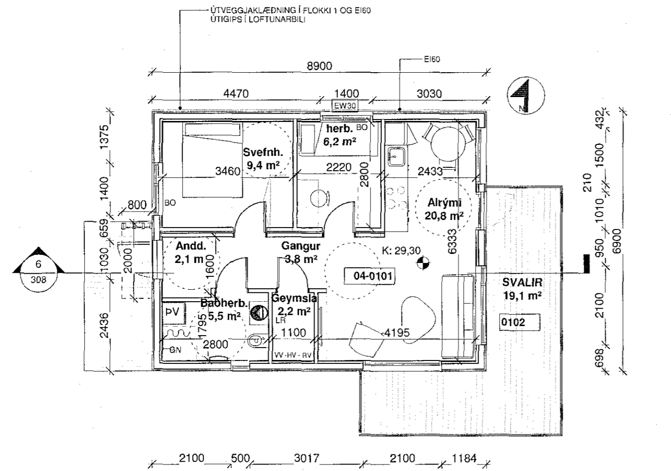
mhl. 04 GRUNNMYND 1:100
