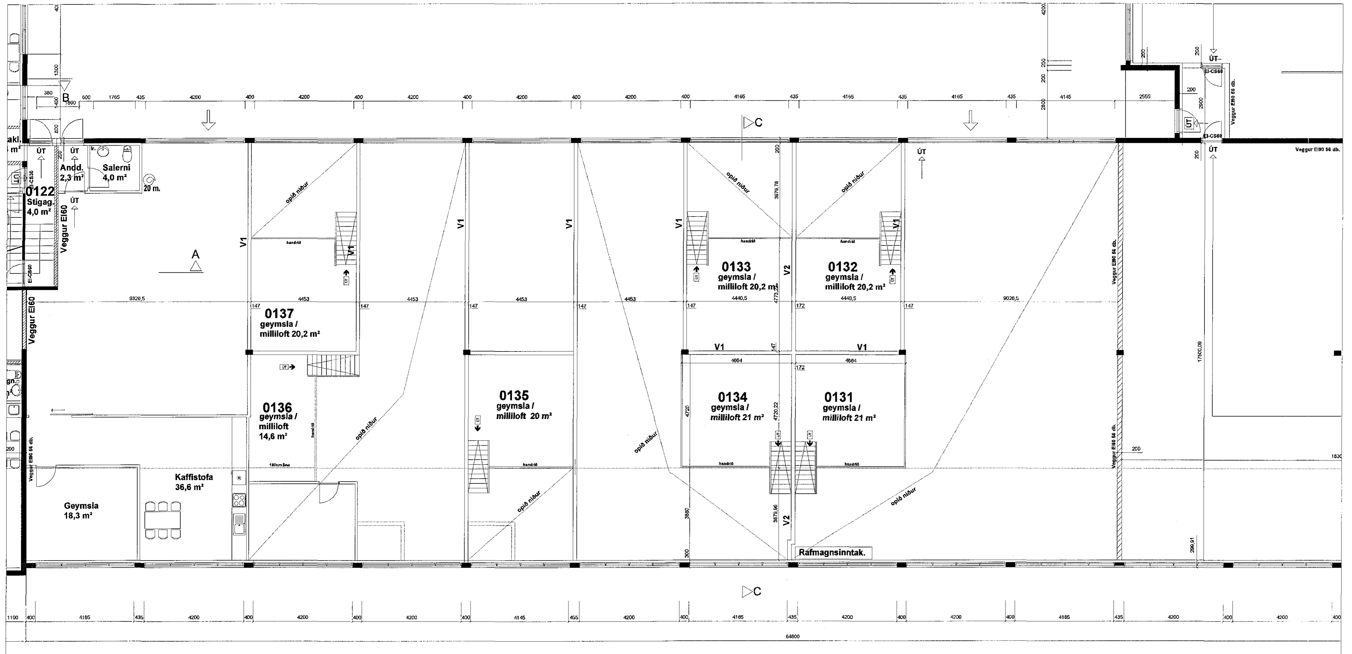
Grunnmynd millilofts mkv 1:100
