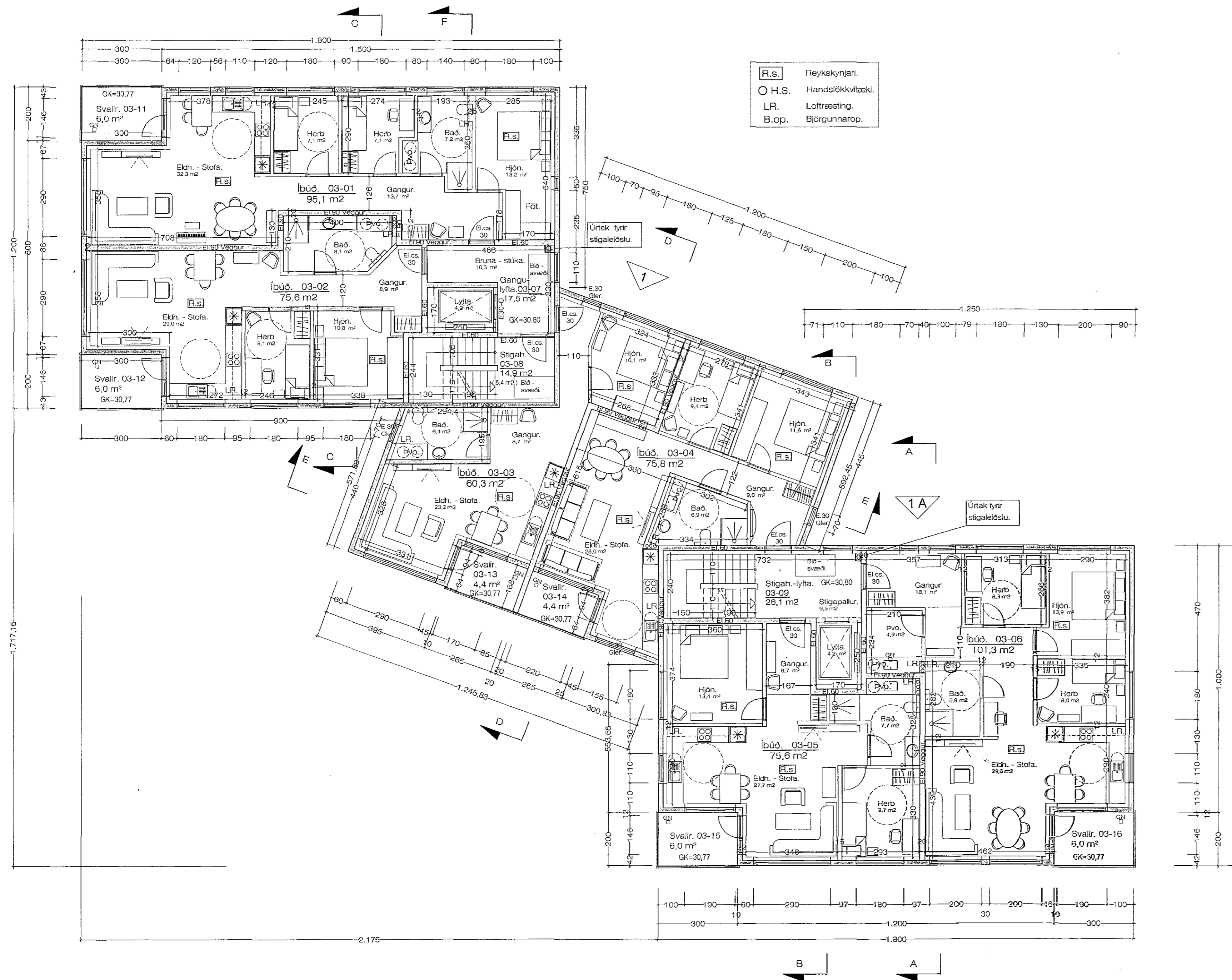
Grunnmynd 3. hæð. 1:100 Stærð. 3. hæðar. 542,2 m 2
