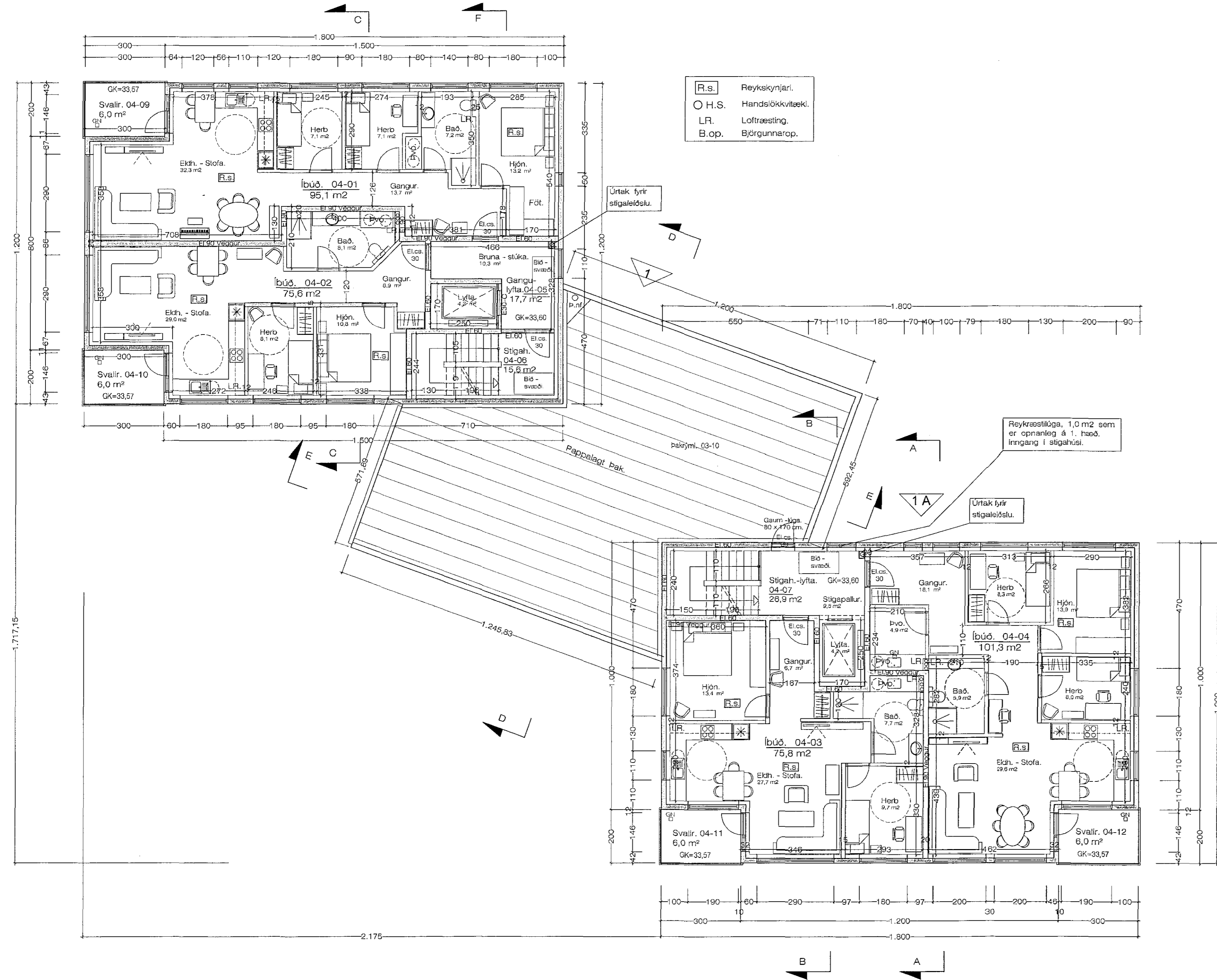
Grunnmynd 4. hæð. 1 : 100 Stærð. 4. hæðar. 408,0 m 2
