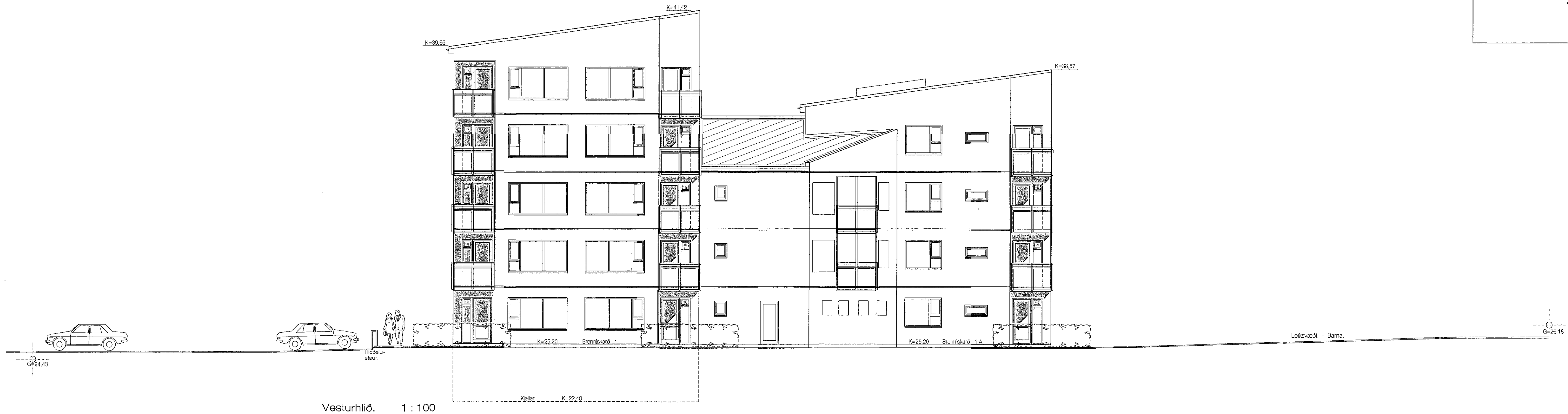
Vesturhlíð. 1 : 100
