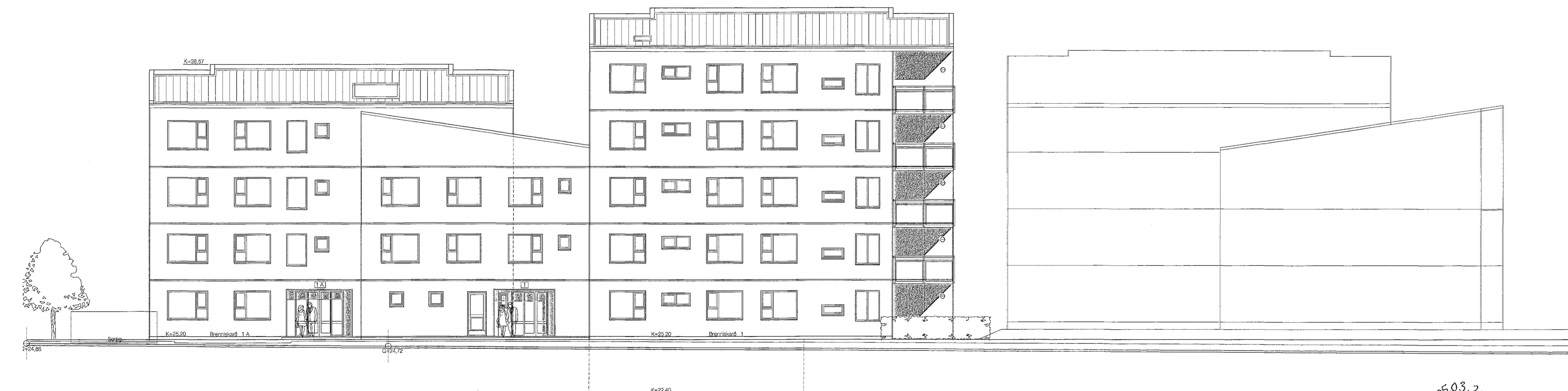
Norðurhlíð. 1 : 100
