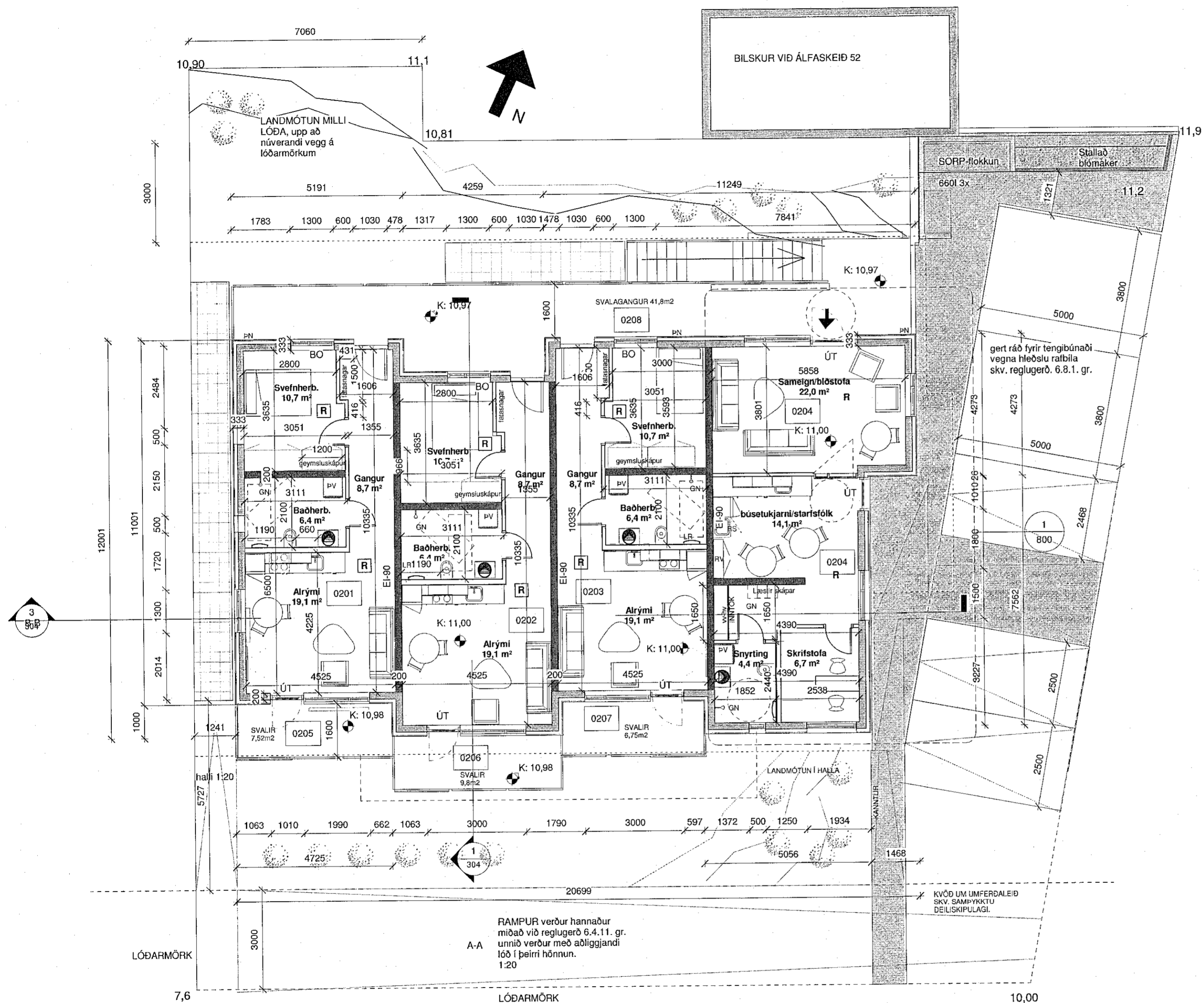
GRUNNMYND 1. HÆÐ 1:100
