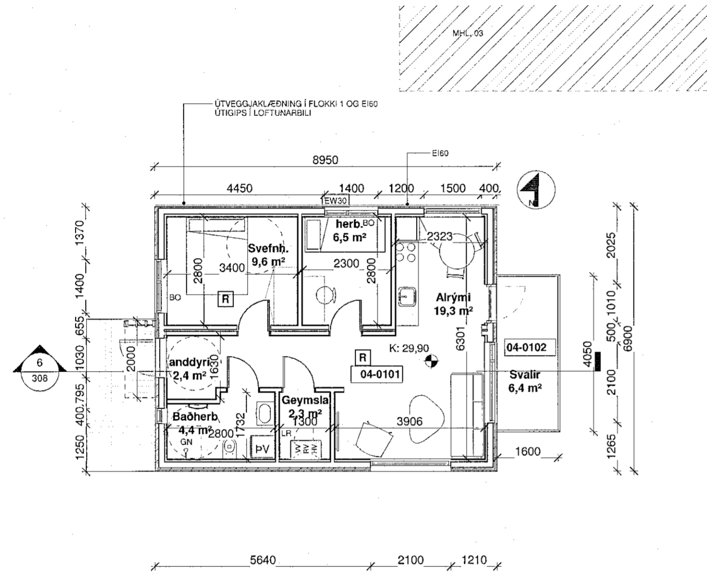
mhl. 04 GRUNNMYND 1 : 100
