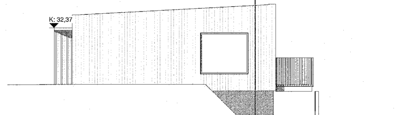
mhl. 04 ásýnd suður. 1 : 100
