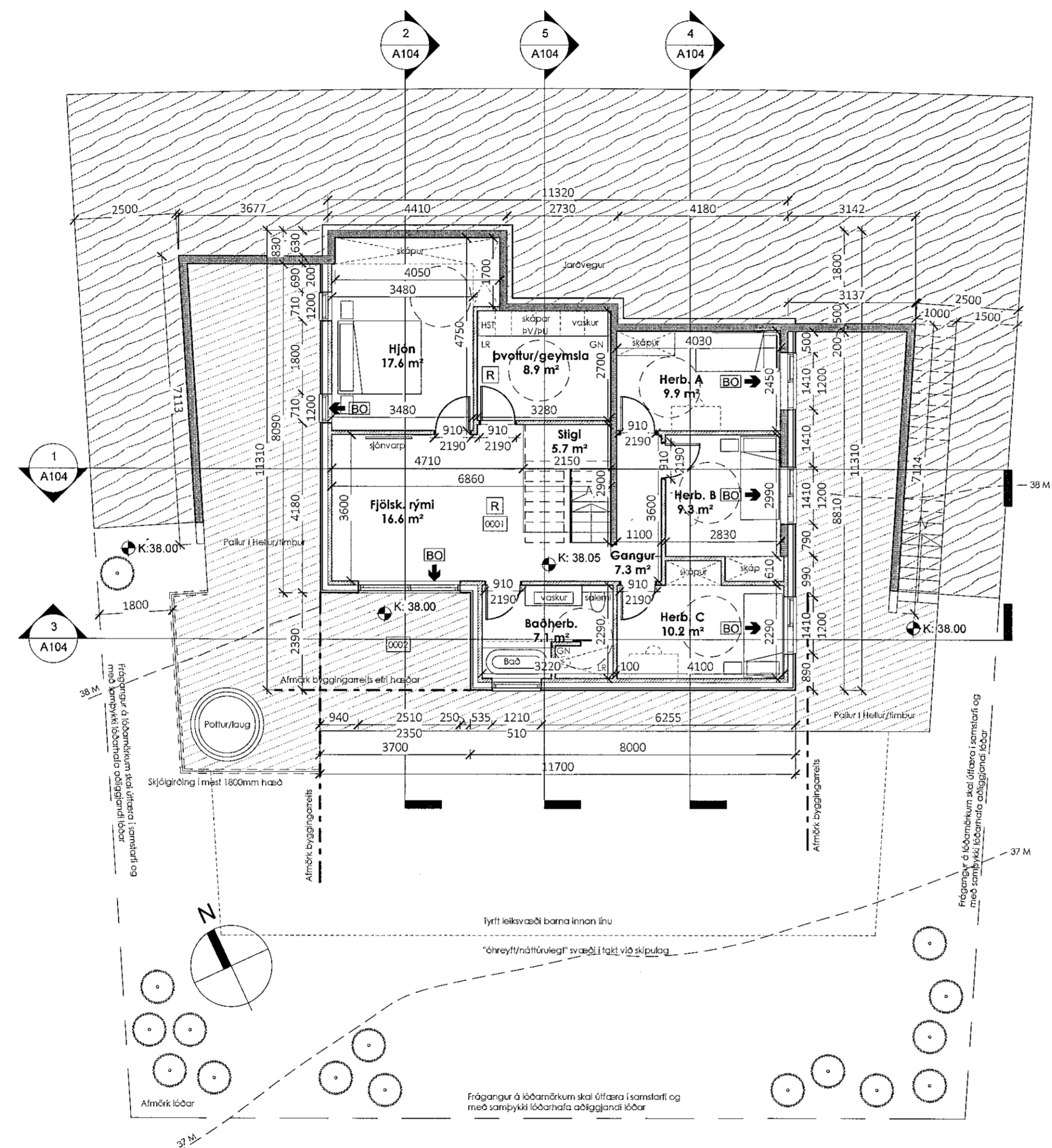
1 00 KJALLARI 1 : 100
