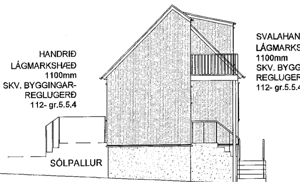
VESTUR MKV. 1:100
