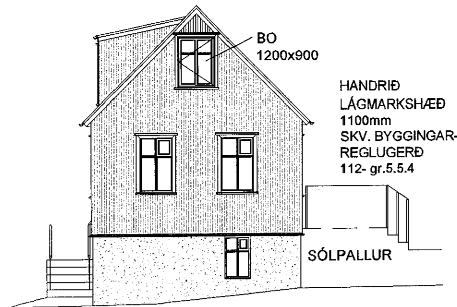
AUSTUR MKV. 1:100
