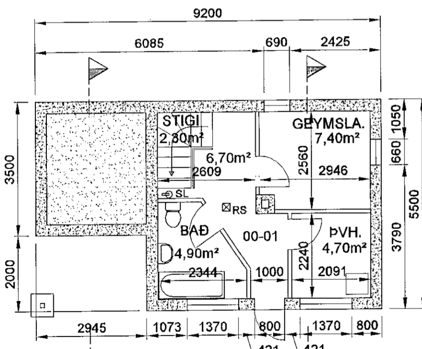
01 - KJALLARI MKV. 1:100
