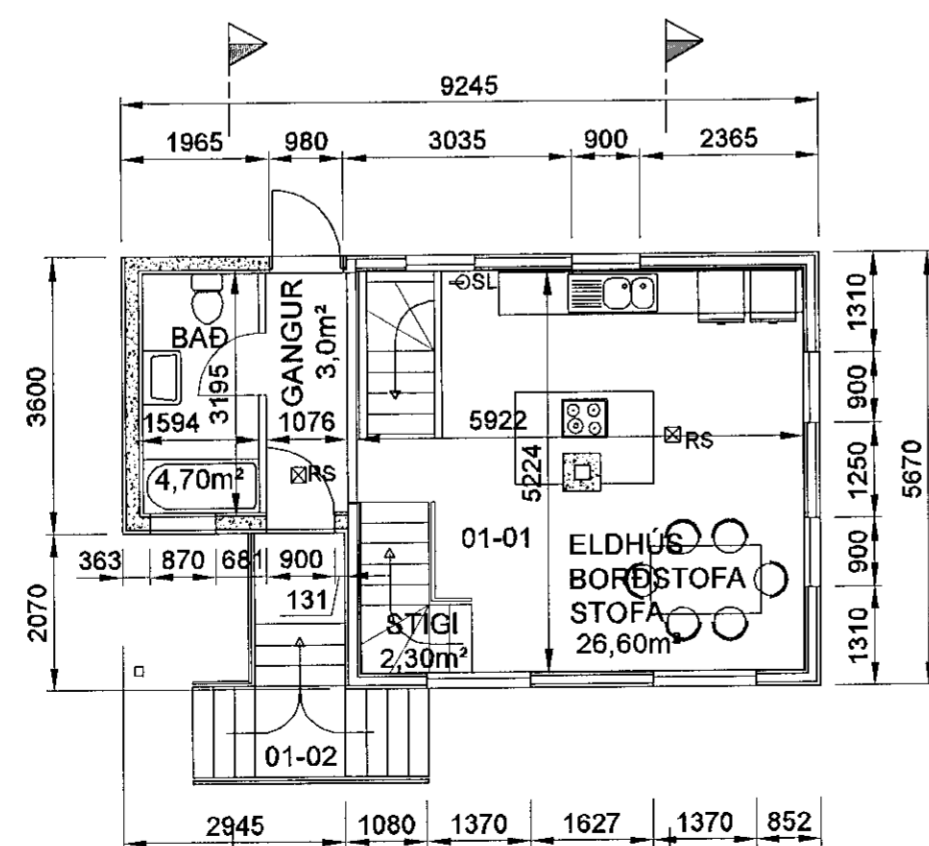
01 - 1. HÆÐ MKV. 1:100
