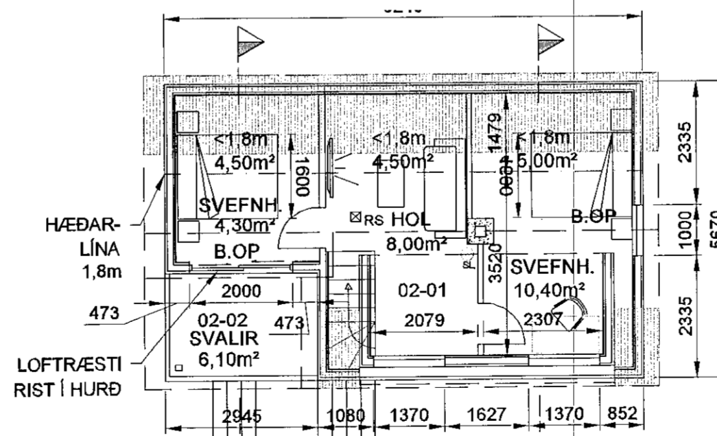
01 - RIS MKV. 1:100
