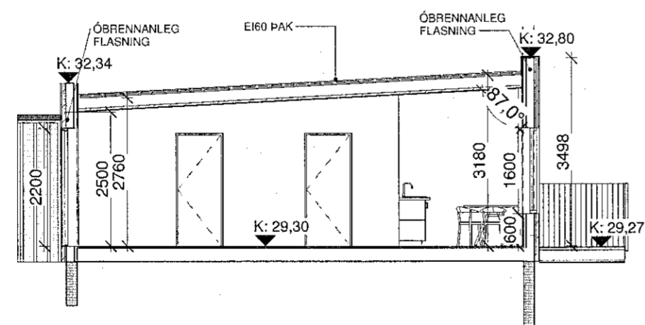
mhl. 04 sneiðing A-A 1 : 100
