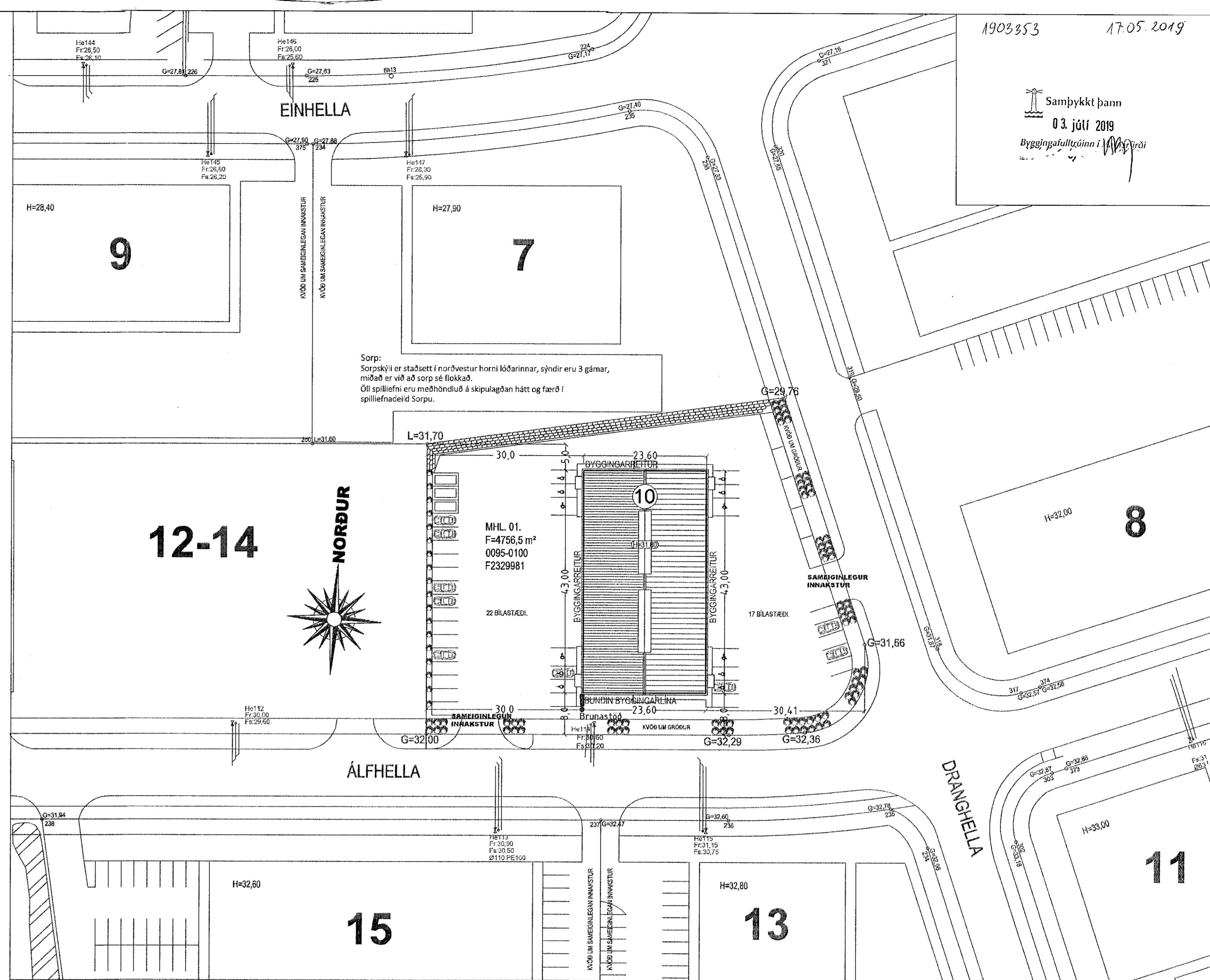
AFSTÖÐUMYND MKV. 1:500.
