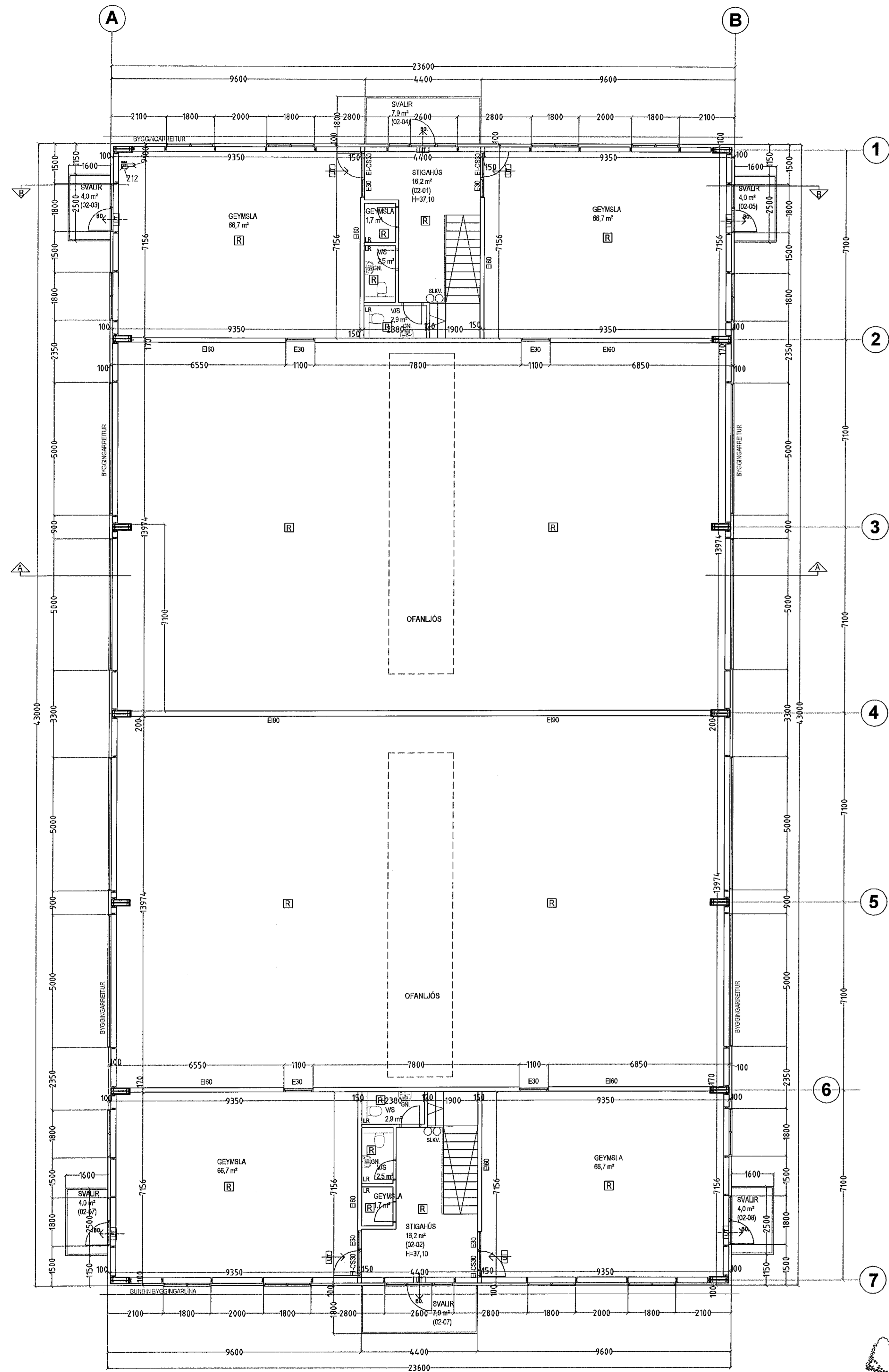
GRUNNMYND 2. HÆÐ MKV. 1:100.
