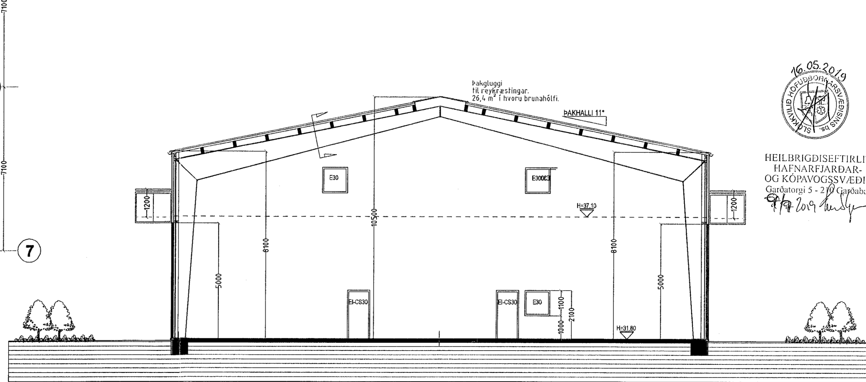
SNIÐ A-A MKV. 1:100.
