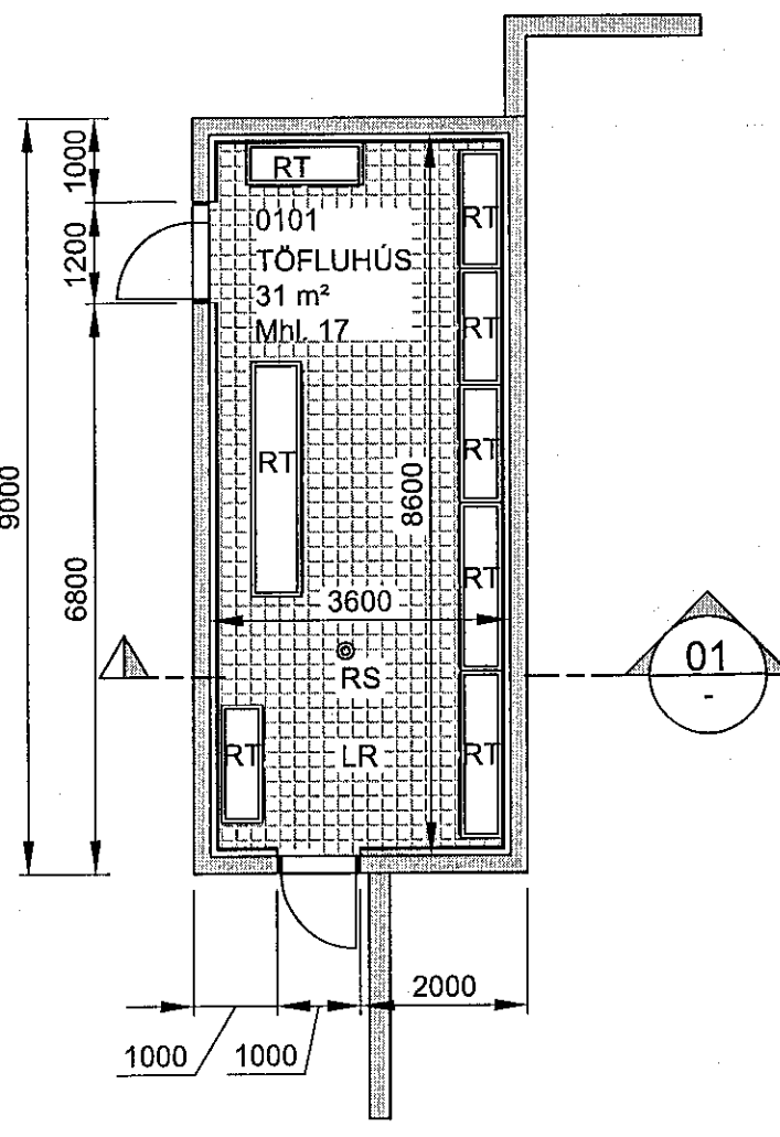
GRUNNMYND TÖFLUHÚSS 1:100
