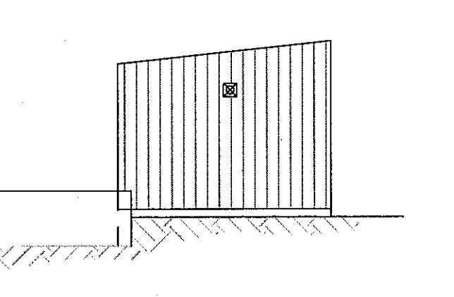
AUSTURHLIÐ 1:100
