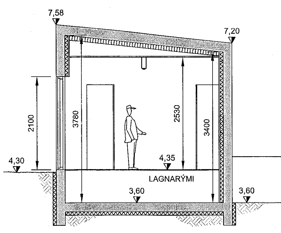
01 SNIÐ 1:50
