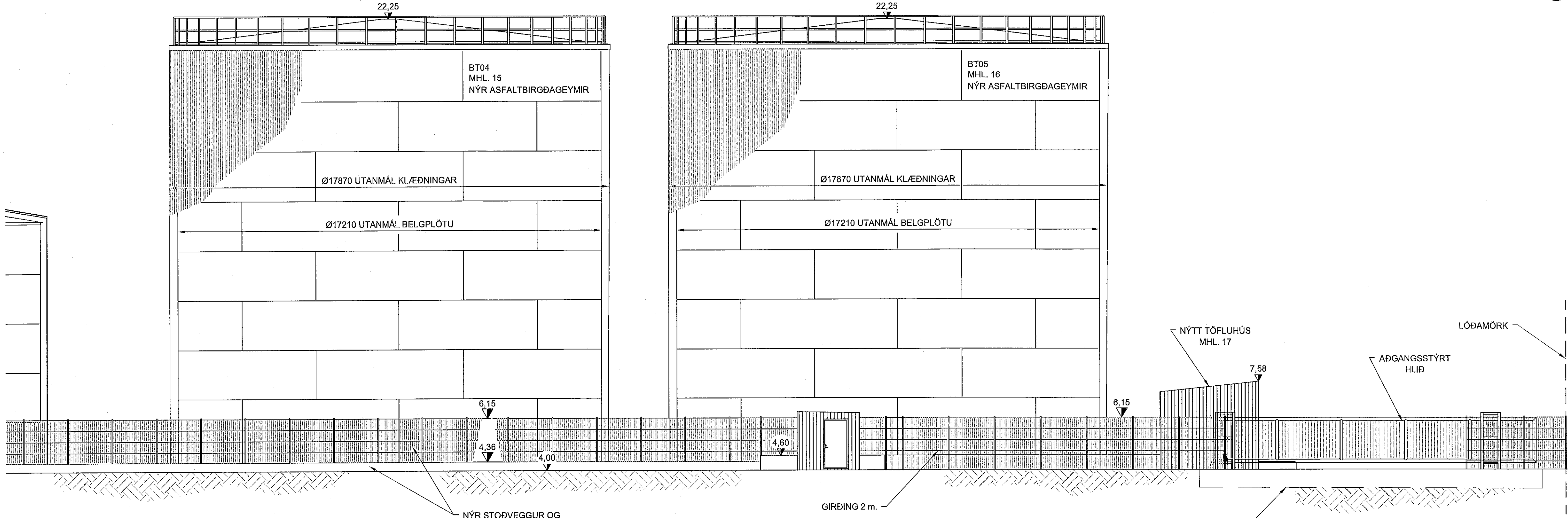
SÉRMYND - (GAMLI HAFNARGARÐURINN EKKI SÝNDUR) 1:100
