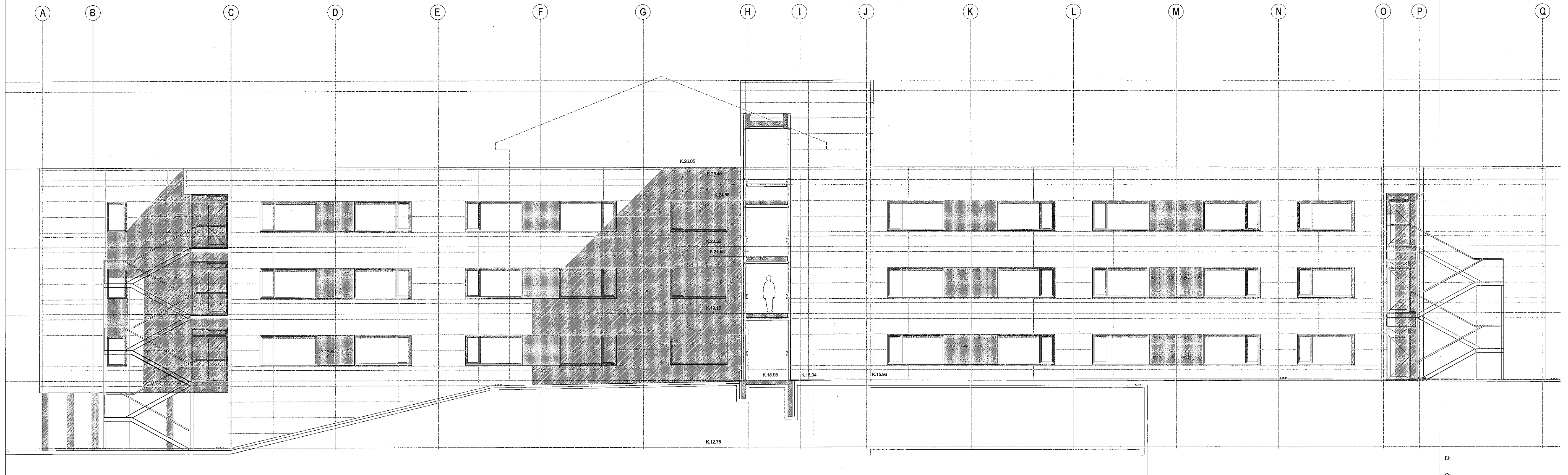
SNEIÐING D-D 1:100
