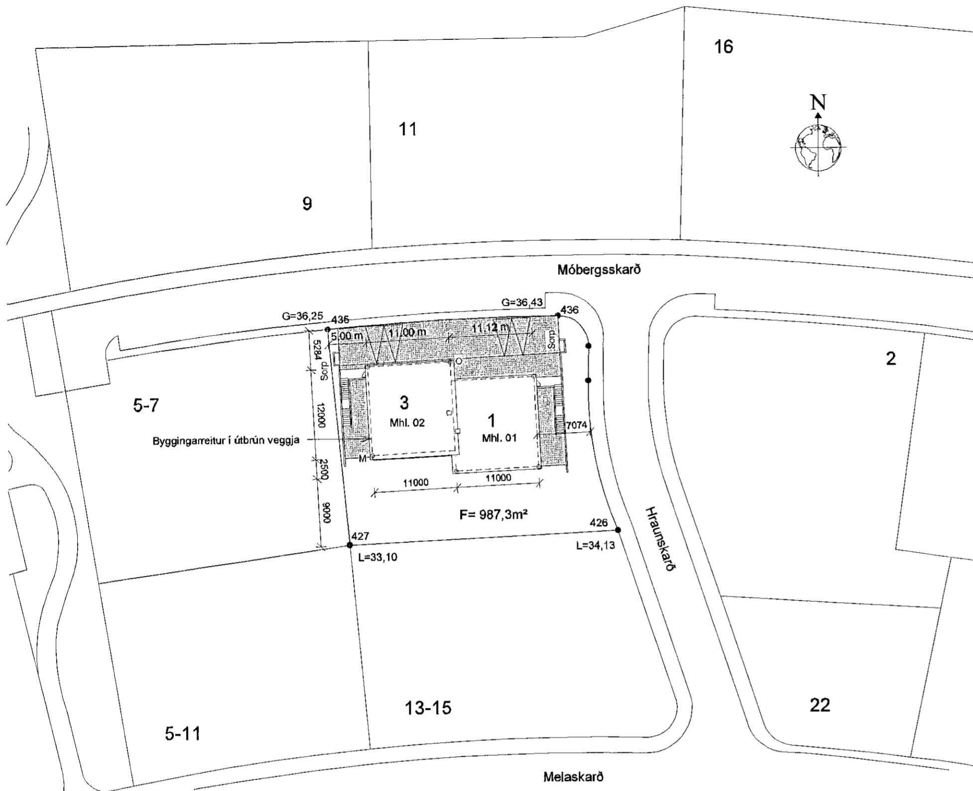
1 Afstöðumynd Mkv. 1: 500
