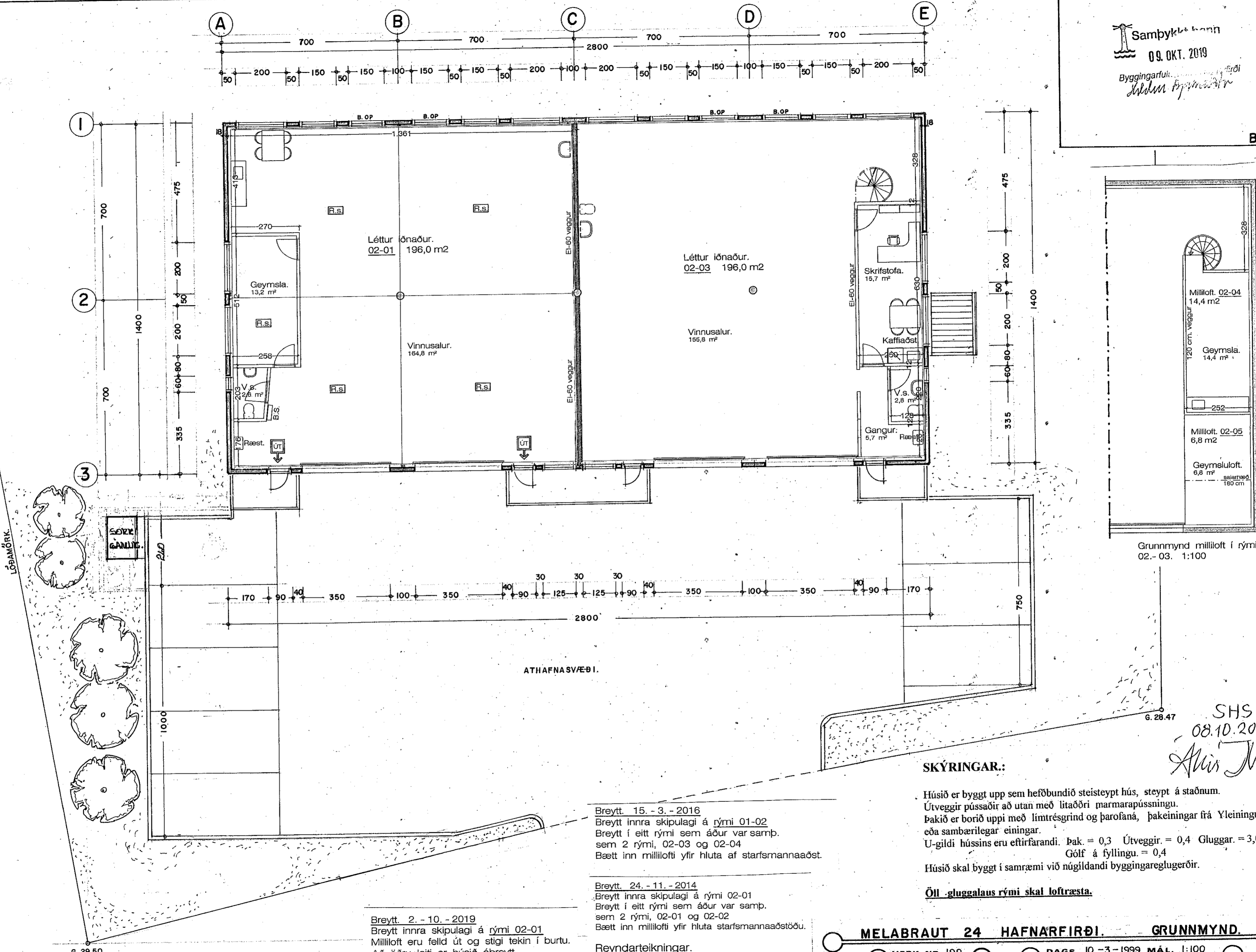
GRUNNMYND. 2. HÆÐ. 1:100
