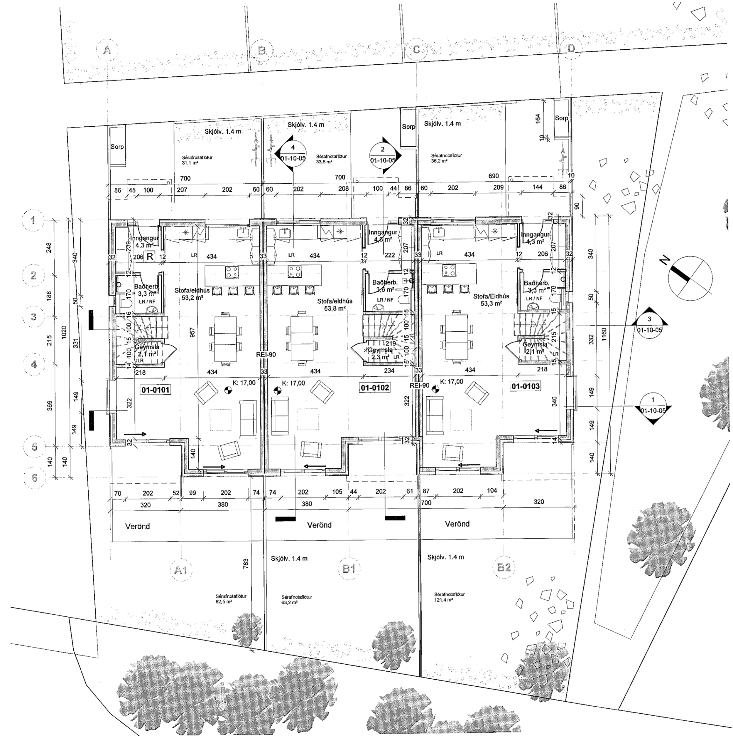
1. hæð (mhl 01) 1 : 100
