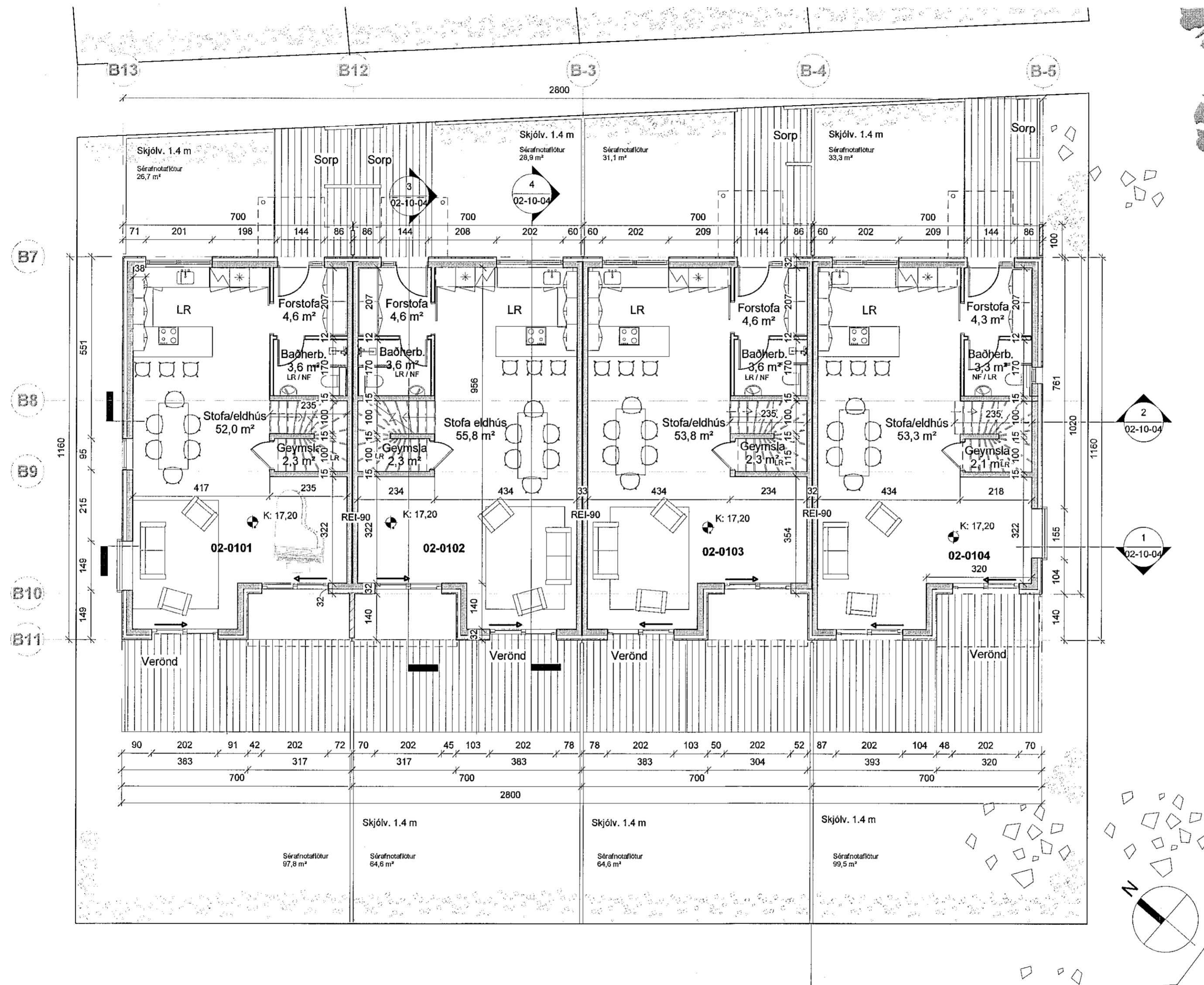
1.hæð (mhl 02) 1 : 100
