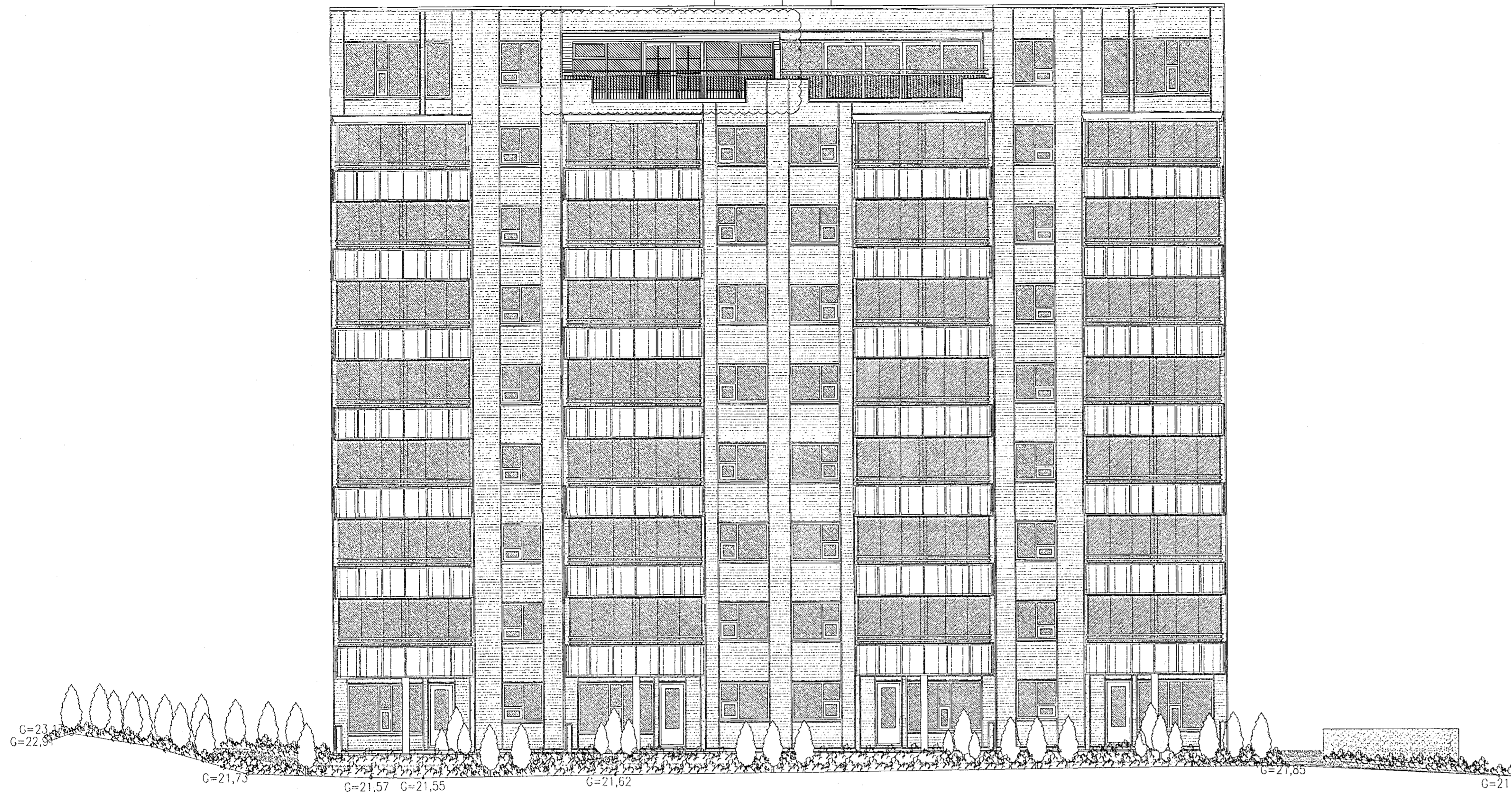
Útlit suður - mkv 1:100
