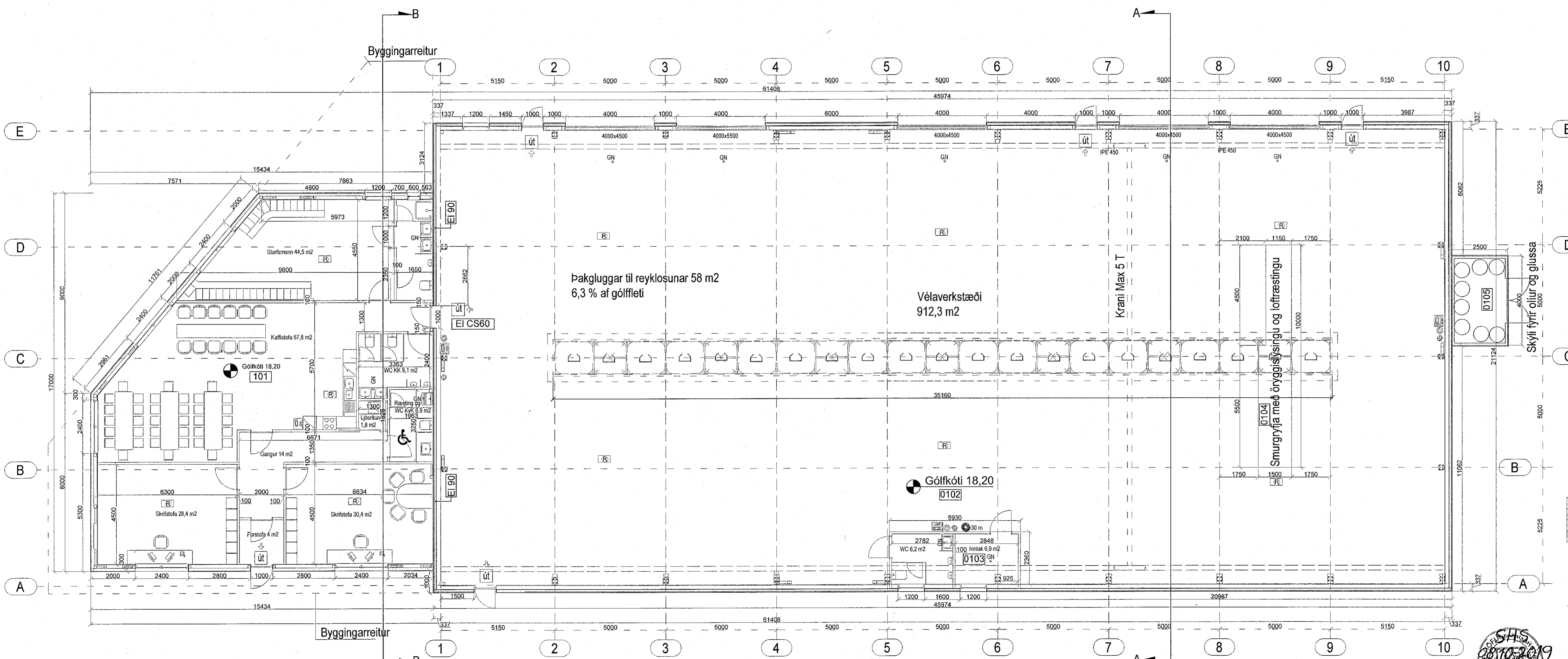
Grunnmynd 1:100
