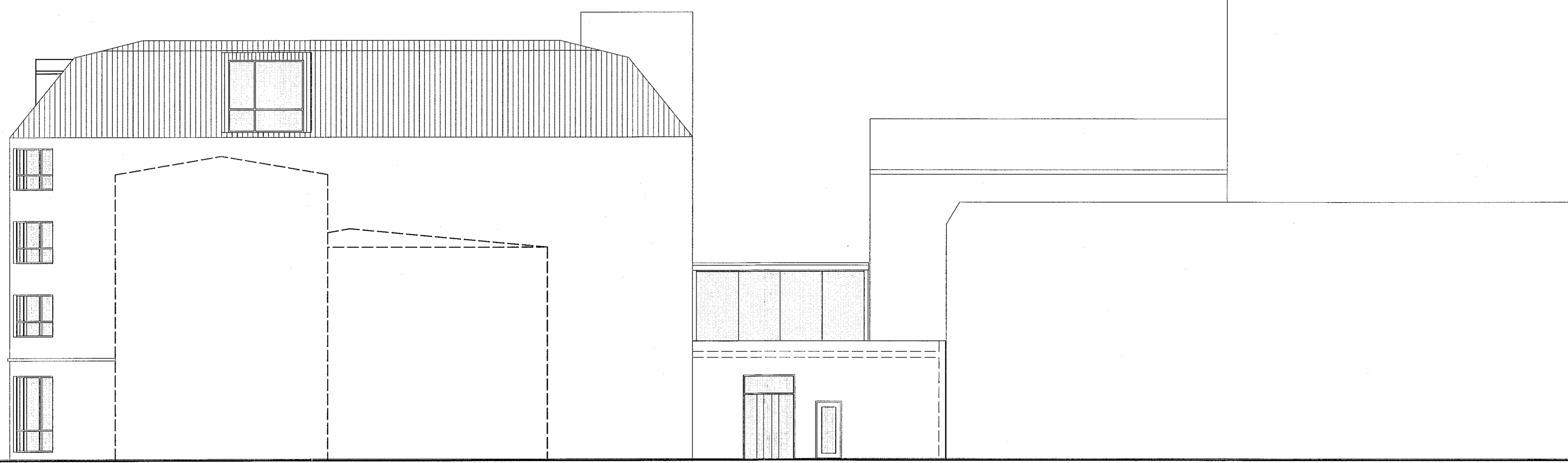
ÚTLIT 1:100 Norð-vestur
