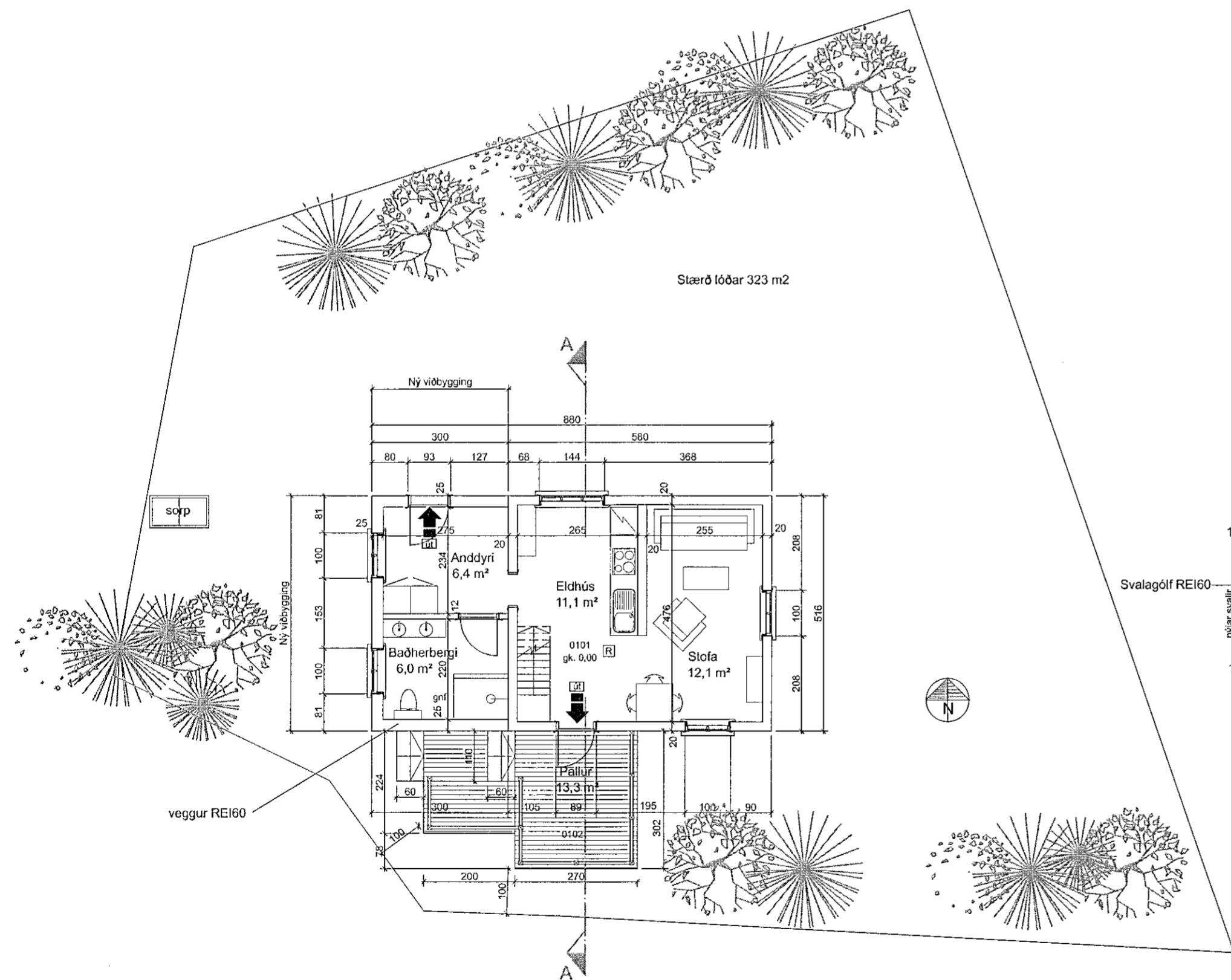
Grunnmynd jarðhæðar 1:100
