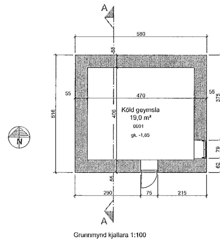
Grunnmynd kjallara 1:100
