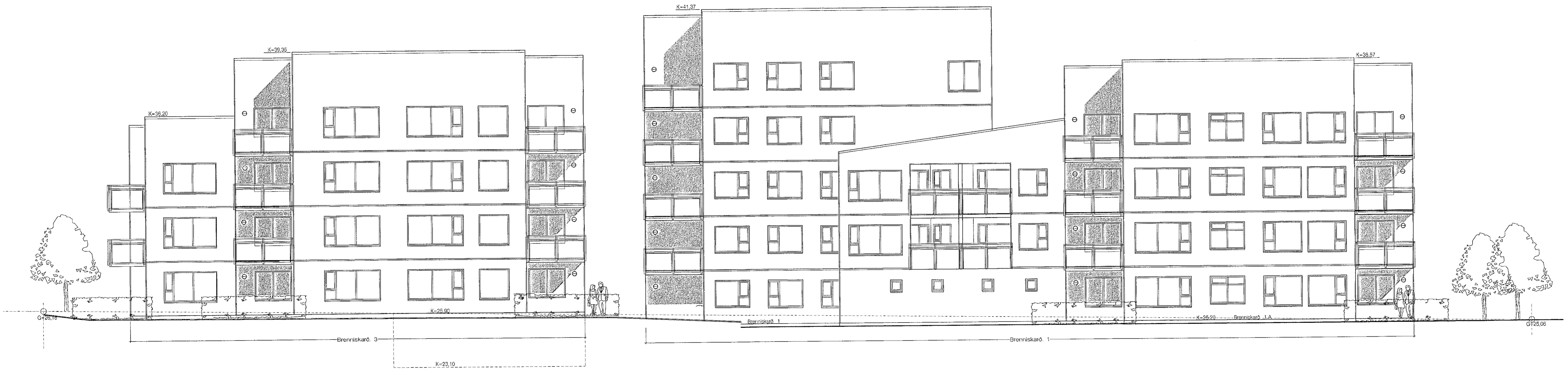
Suðurhlíð. 1 : 100
