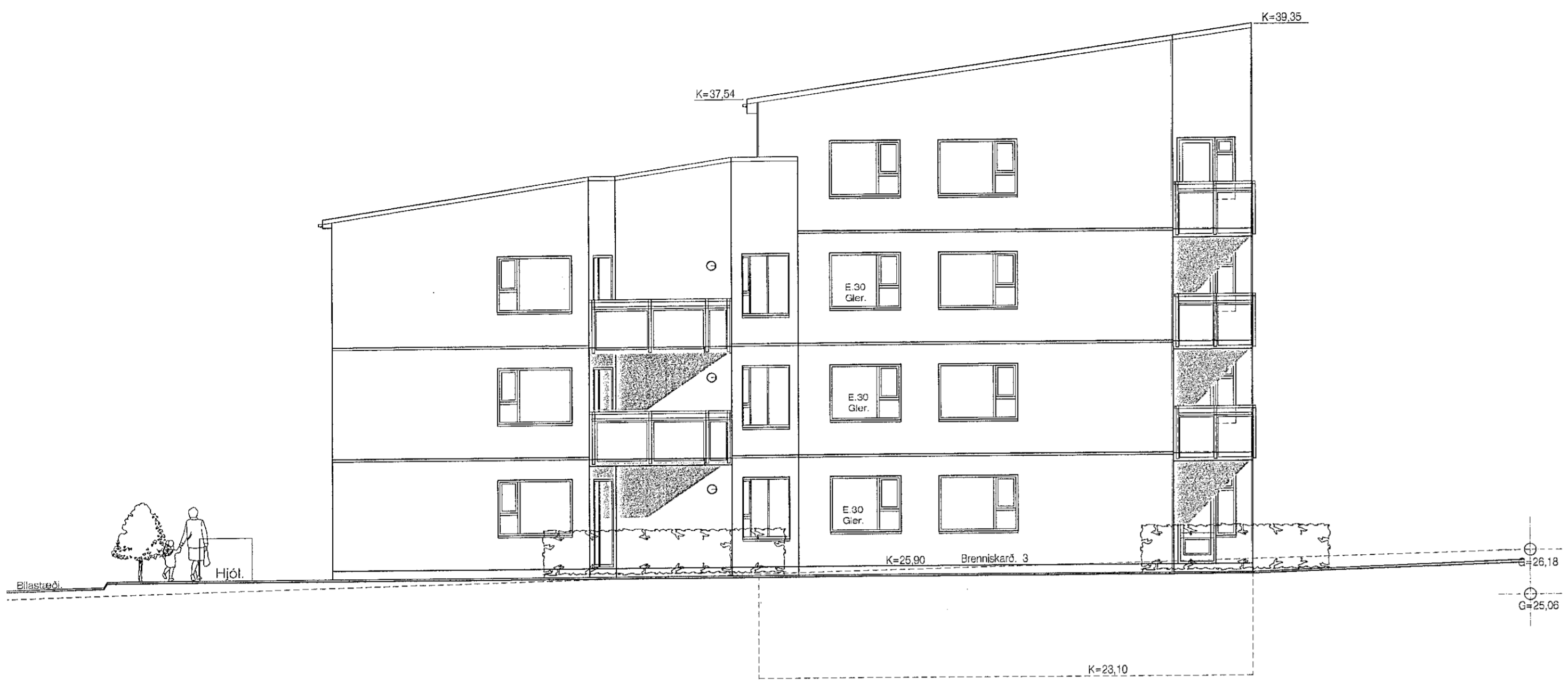
Vesturhlíð. 1 : 100
