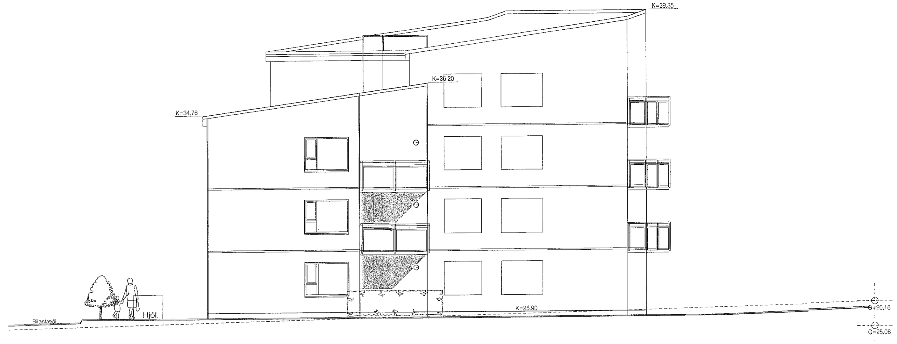
Norð - Vesturhlíð. 1 : 100
