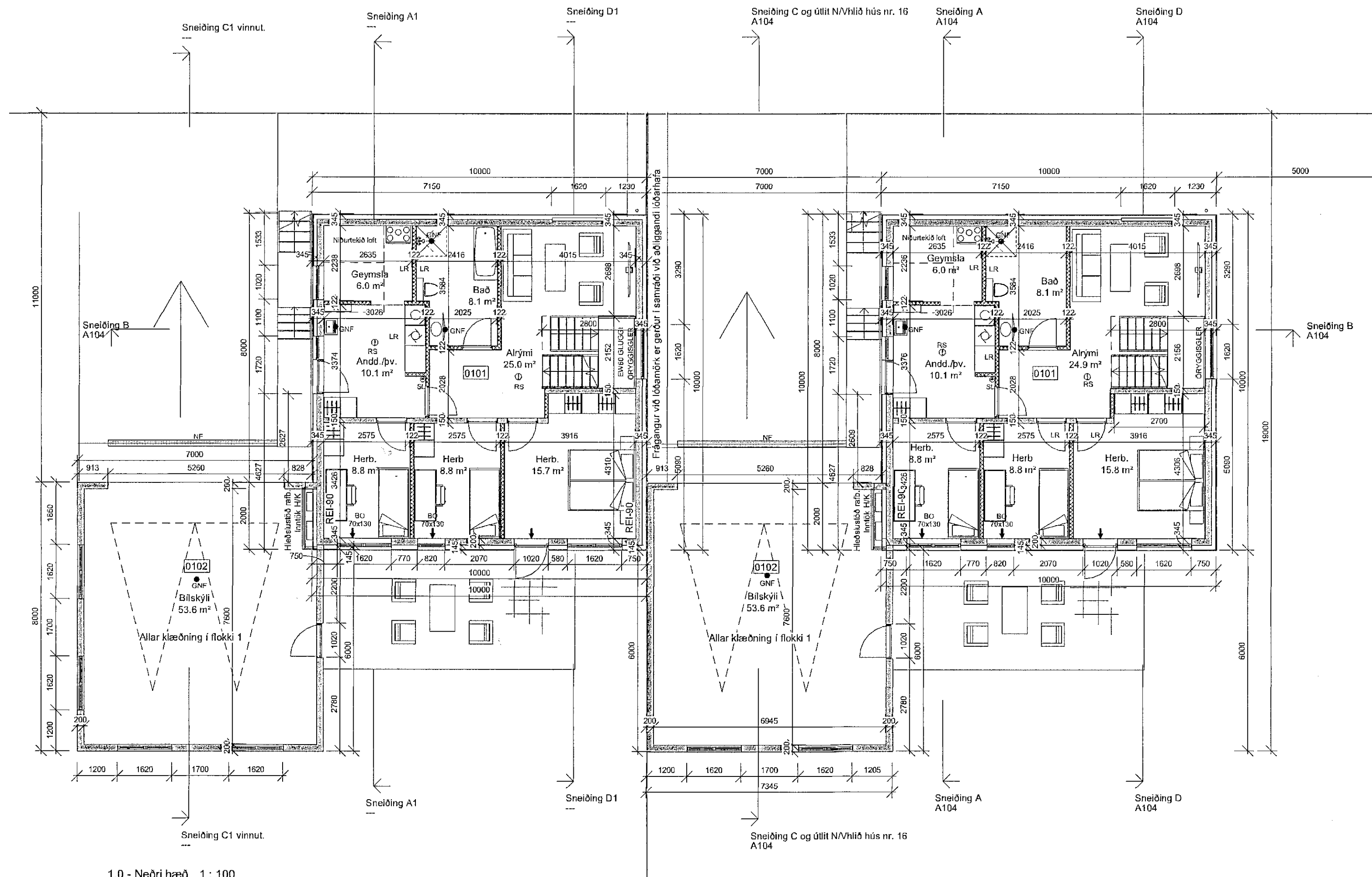
1.0 - Neðri hæð 1 : 100
