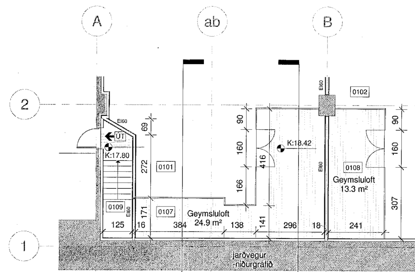
1. hæð, millioft 1:100
