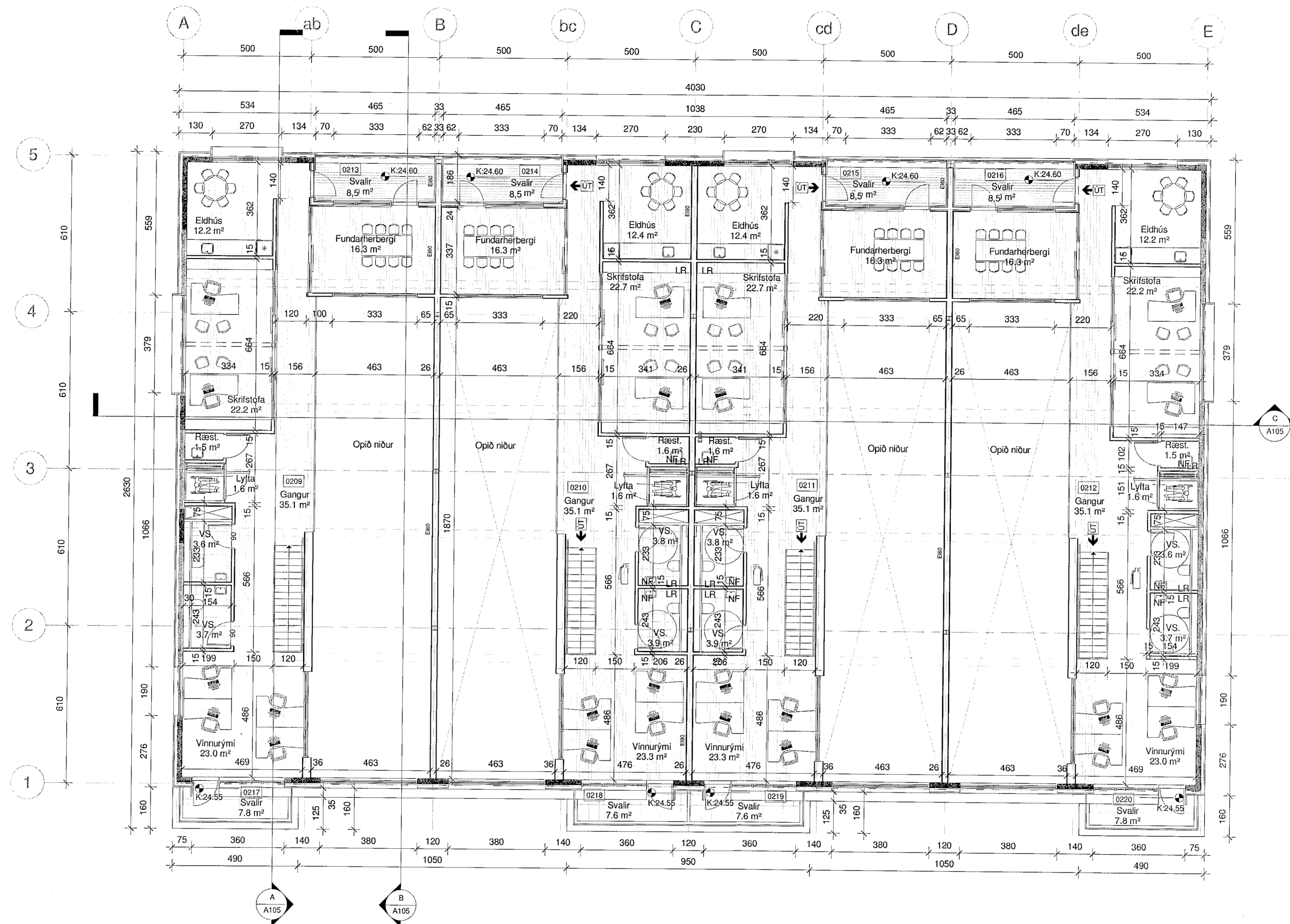
2. hæð, millifletir 1:100
